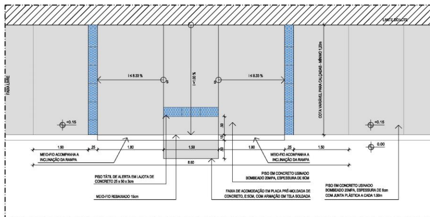
Figura 4 - Rampa para o acesso de pedestres - TIPO B
