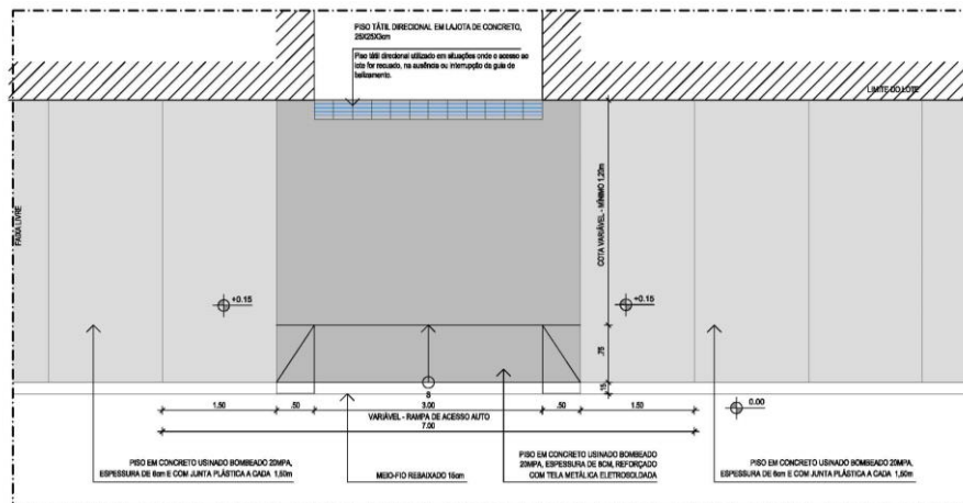
Figura 5 - Rampa padrão para o acesso de veículos
