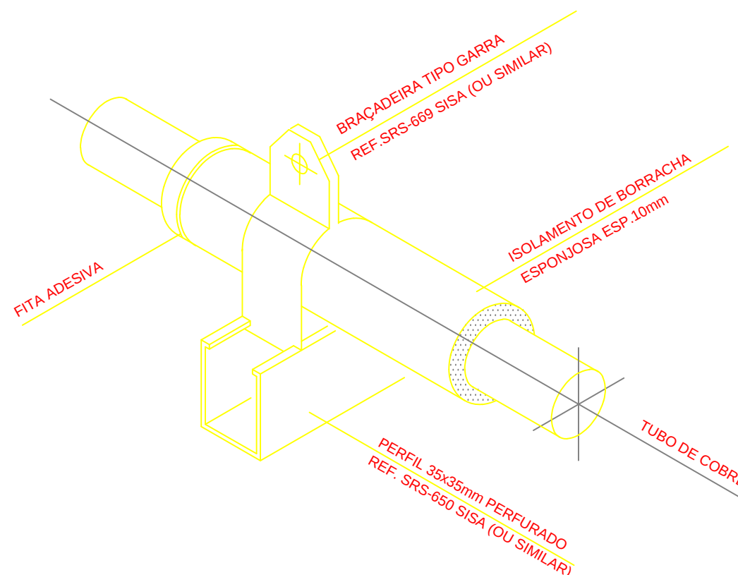
DETALHE 04 - ISOLAMENTO DE TUBOS DE COBRE INTERNOS Sem Escala
