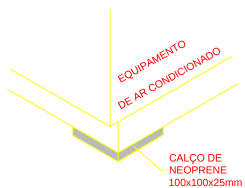
DETALHE 03 - CALÇO PARA CONDENSADORAS Sem Escala
