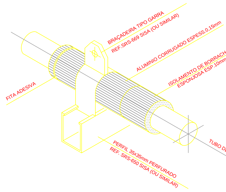
DETALHE 05 - ISOLAMENTO DE TUBOS DE COBRE EXTERNOS Sem Escala
