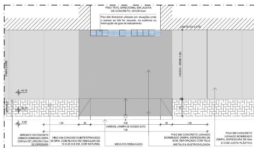
Figura 3 - Rampa padrão para o acesso de veículos
