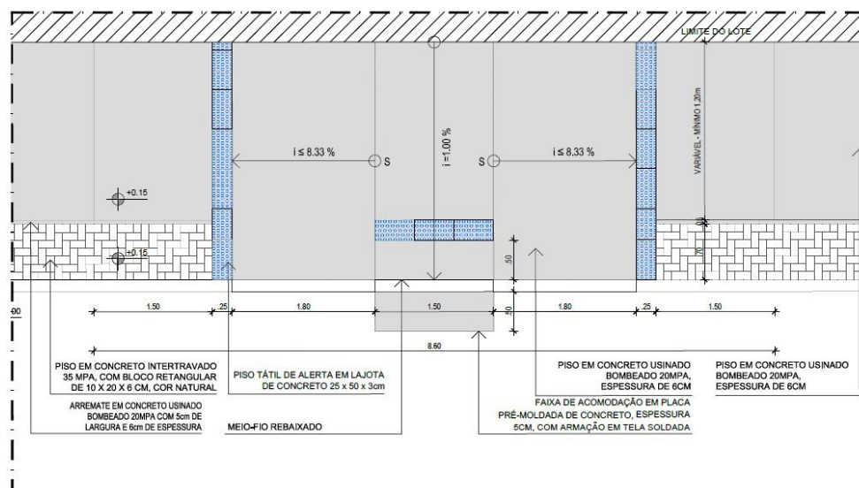
Figura 2 - Rampa para o acesso de pedestres - TIPO B
