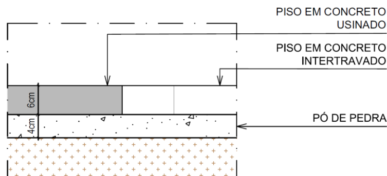
Figura 14 - Seção Tipo de Pavimentação
