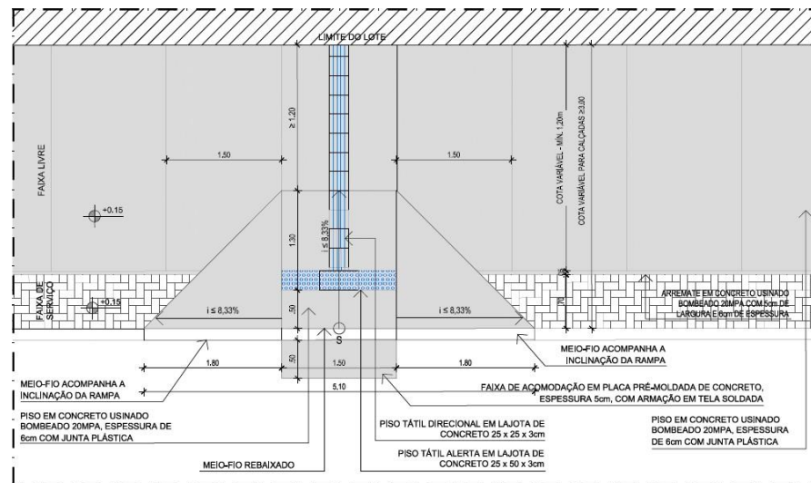
Figura 1 - Rampa para o acesso de pedestres - TIPO A
