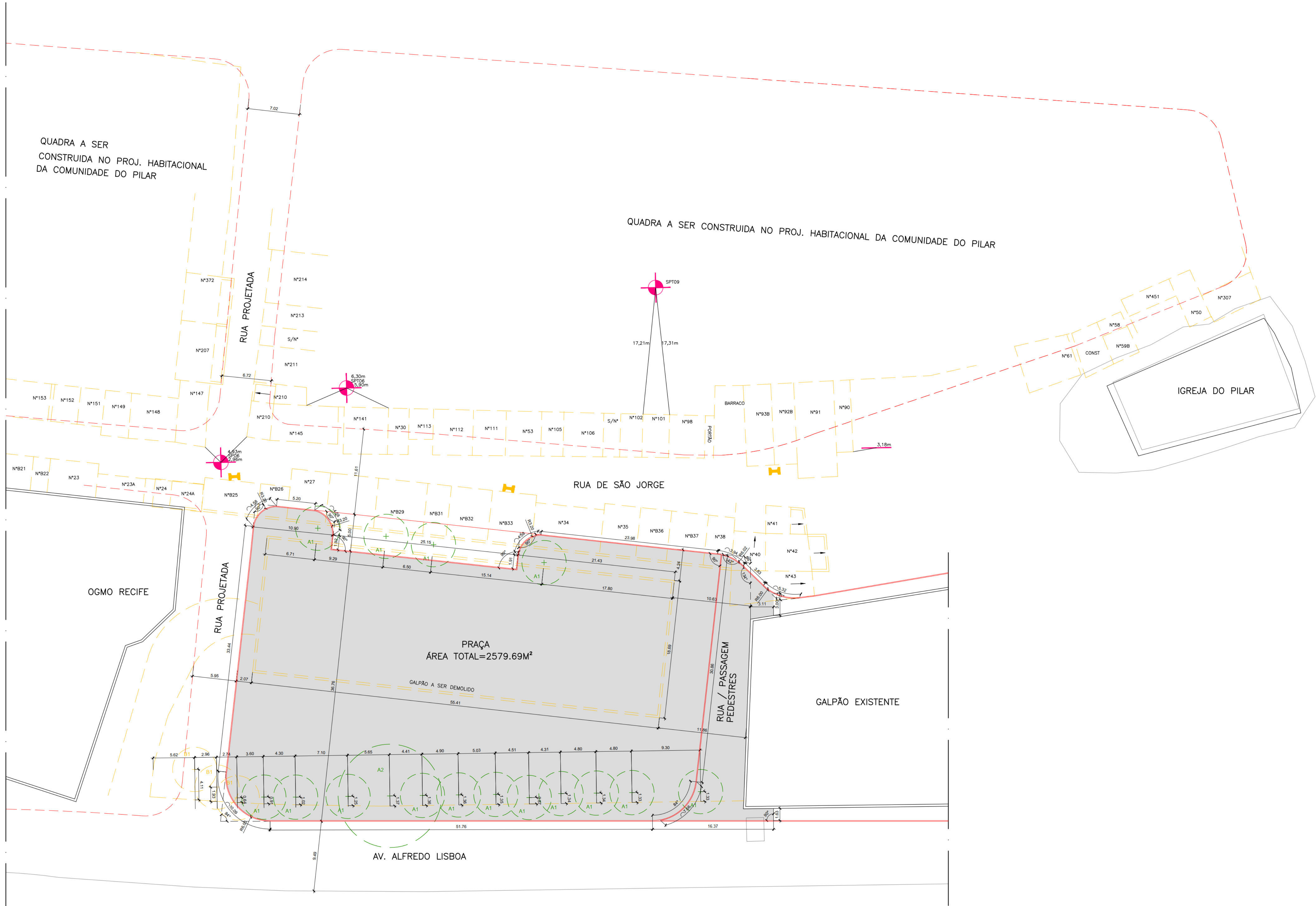
PLANTA DE DEMOLIÇÃO E CONSTRUÇÃO (PLANTA DE SITUAÇÃO EXISTENTE) ESC.: 1/250
