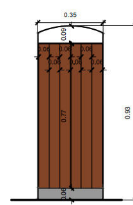
DETALHE LIXEIRA (elevação frontal) Escala 1:20
