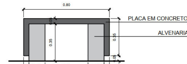
DETALHE BANCO CONCRETO (corte) Escala 1:20
