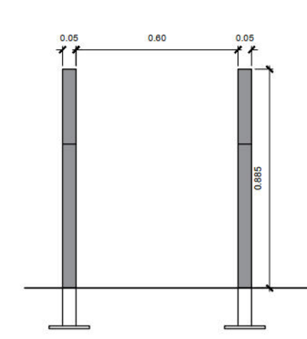
DETALHE BICICLETÁRIO (elevação frontal) Escala 1:20
