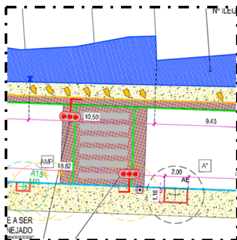
Figura 7 – Proposta de criação de faixa elevada para travessia de pedestre na Rua Ladeira de Pedra
