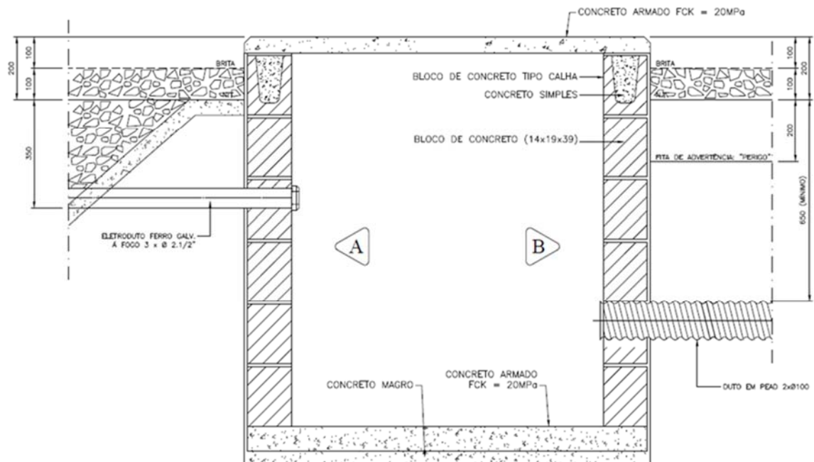
Figura 20 - Alternativa 01 - embutimento completo, corte transversal
