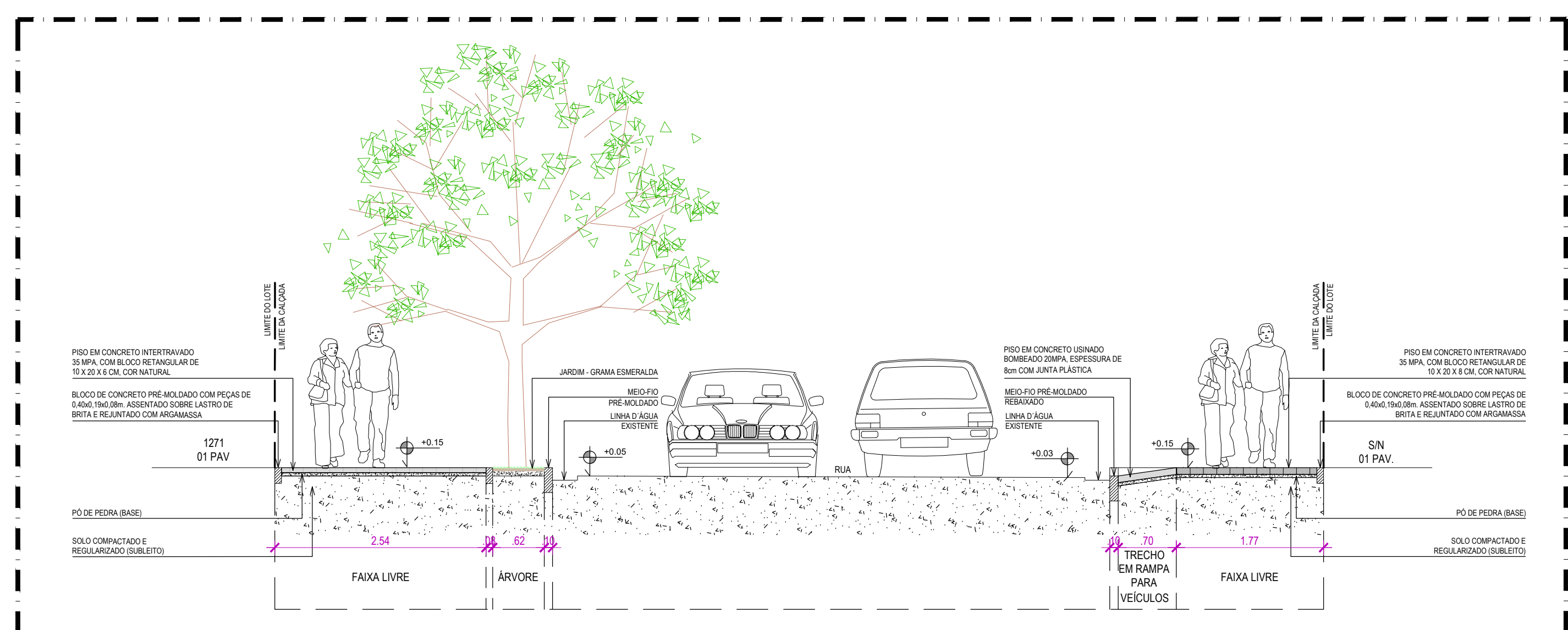
03 CORTE AA' PROPOSTA - TRECHO 01 - VN73 - RUA LADEIRA DE PEDRA
