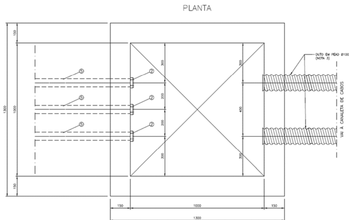
Figura 19 - Alternativa 01 - embutimento completo, Planta
