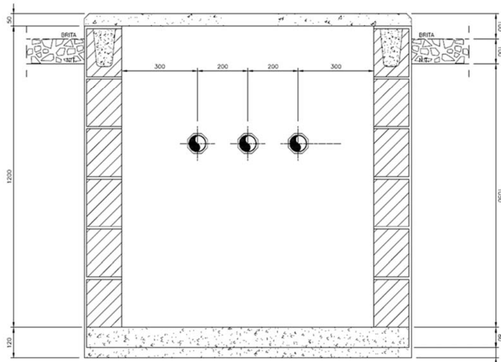
Figura 21 - Alternativa 01 - embutimento completo, corte A
