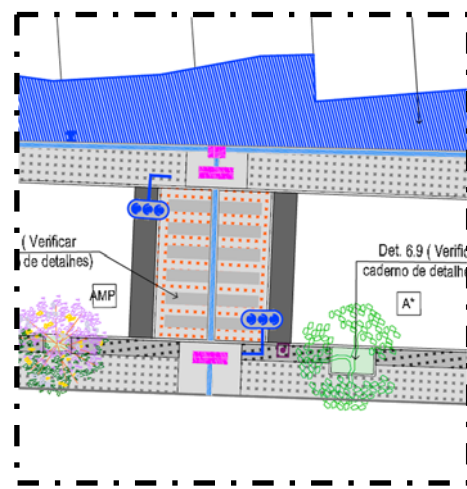
Figura 7 – Proposta de criação de faixa elevada para travessia de pedestre na Rua Ladeira de Pedra
