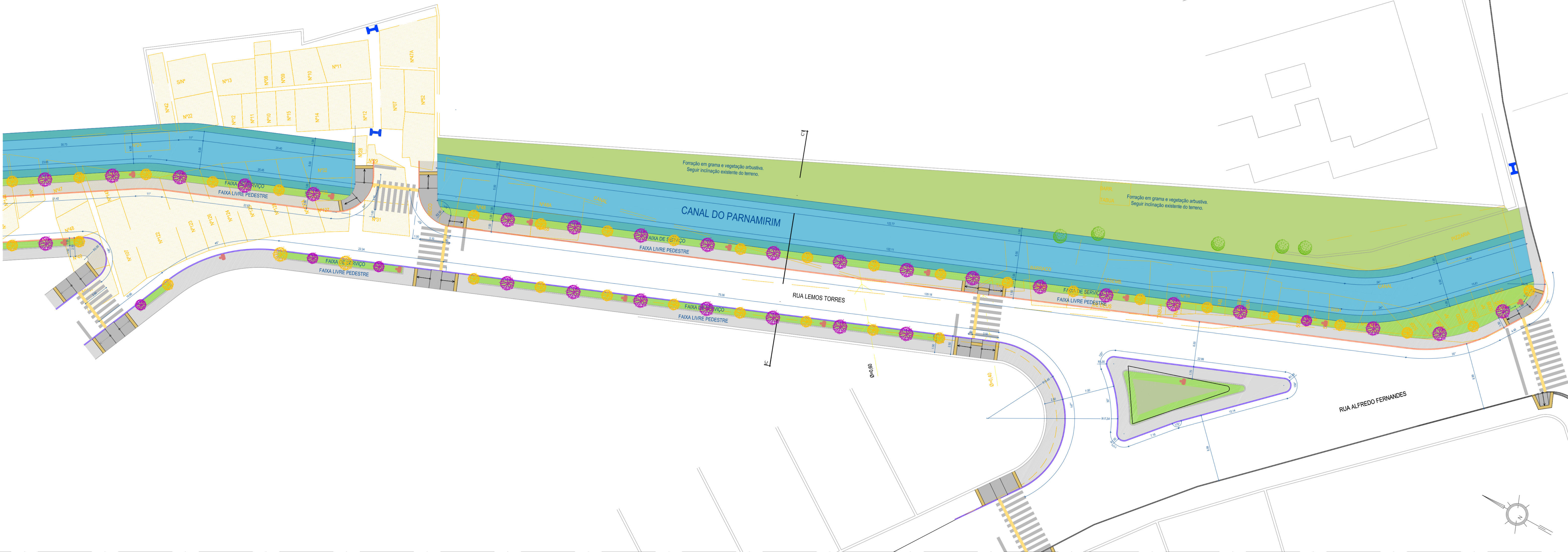
PAISAGISMO - CANAL DO PARNAMIRIM TRECHO 1 ESCALA 1/200
