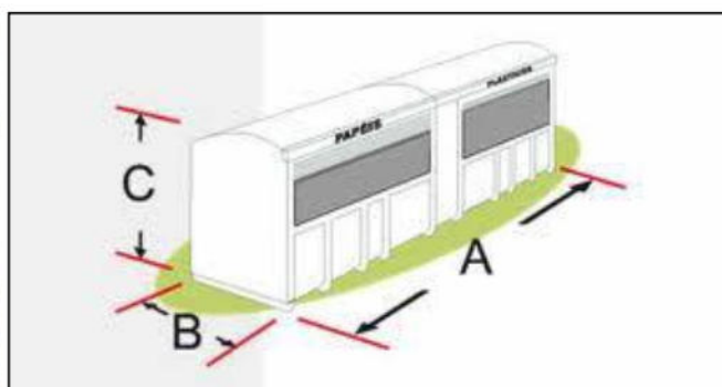
Figura 2 – Modelo de baías utilizadas para o armazenamento final de alguns resíduos no canteiro de obras
