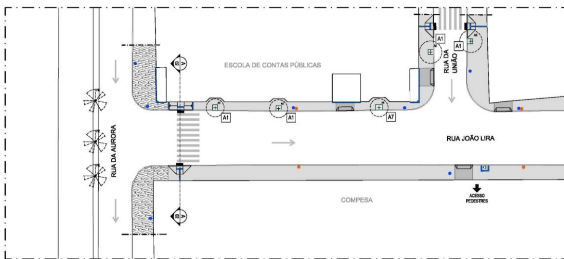
Planta Baixa proposta – Trecho de desvio no gradil da Escola de Contas Públicas e recuo do muro da COMPESA
