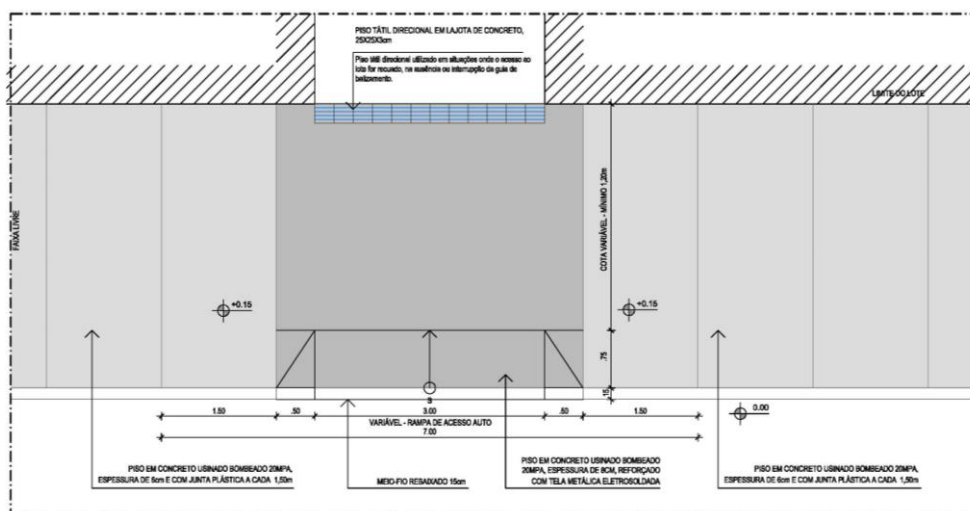
Figura 6 - Rampa padrão para o acesso de veículos
