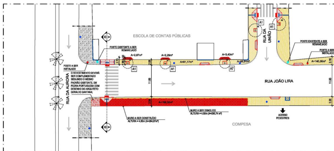
Planta Baixa reforma – Trecho de desvio no gradil da Escola de Contas Públicas e recuo do muro da COMPESA
