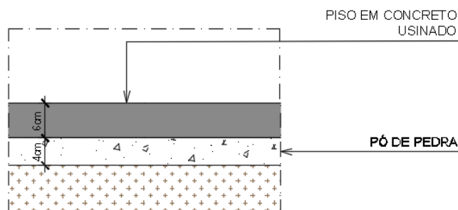
Figura 15 - Seção Tipo de Pavimentação
