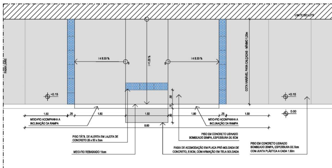
Figura 5 - Rampa para o acesso de pedestres - TIPO B
