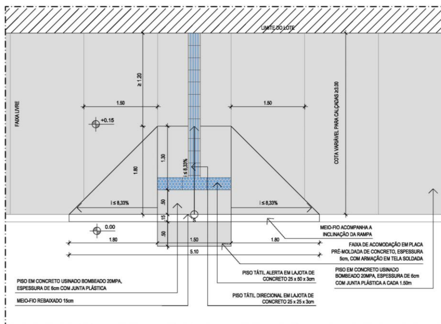
Figura 4 - Rampa para o acesso de pedestres - TIPO A
