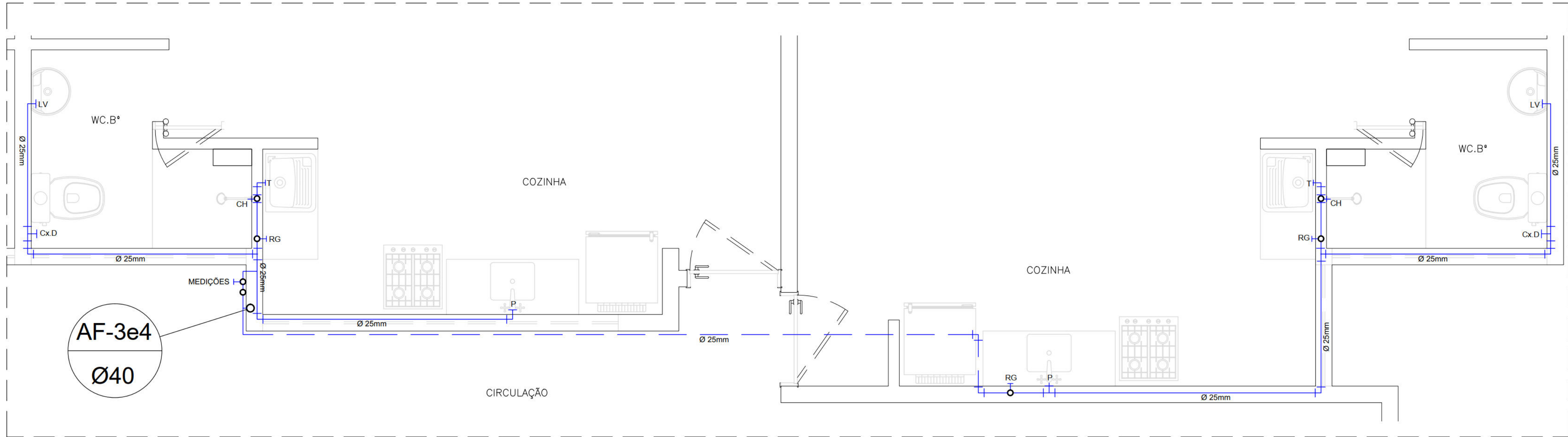
DETALHE 2 ( PLANTA BAIXA ) ESCALA: 1/25
