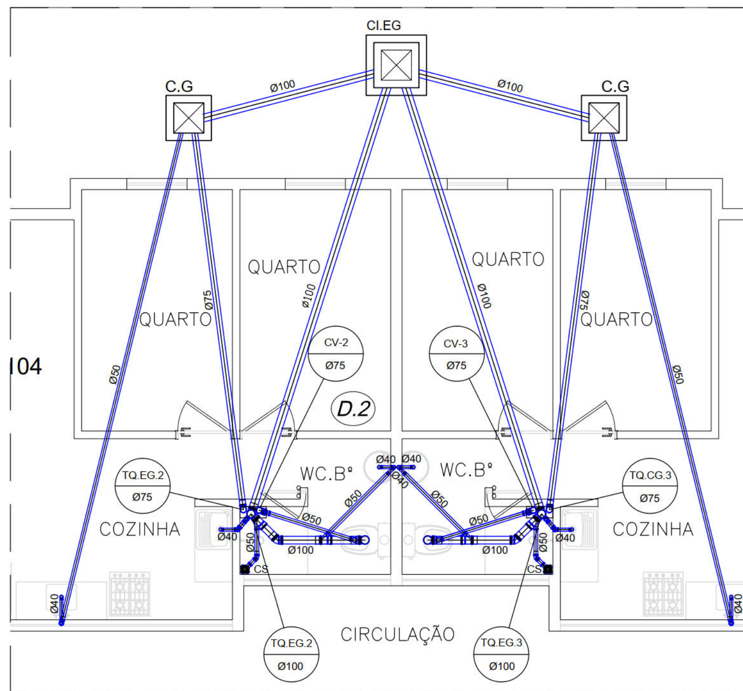
PLANTA BAIXA ESGOTO - TÉRREO ESCALA: 1/25
