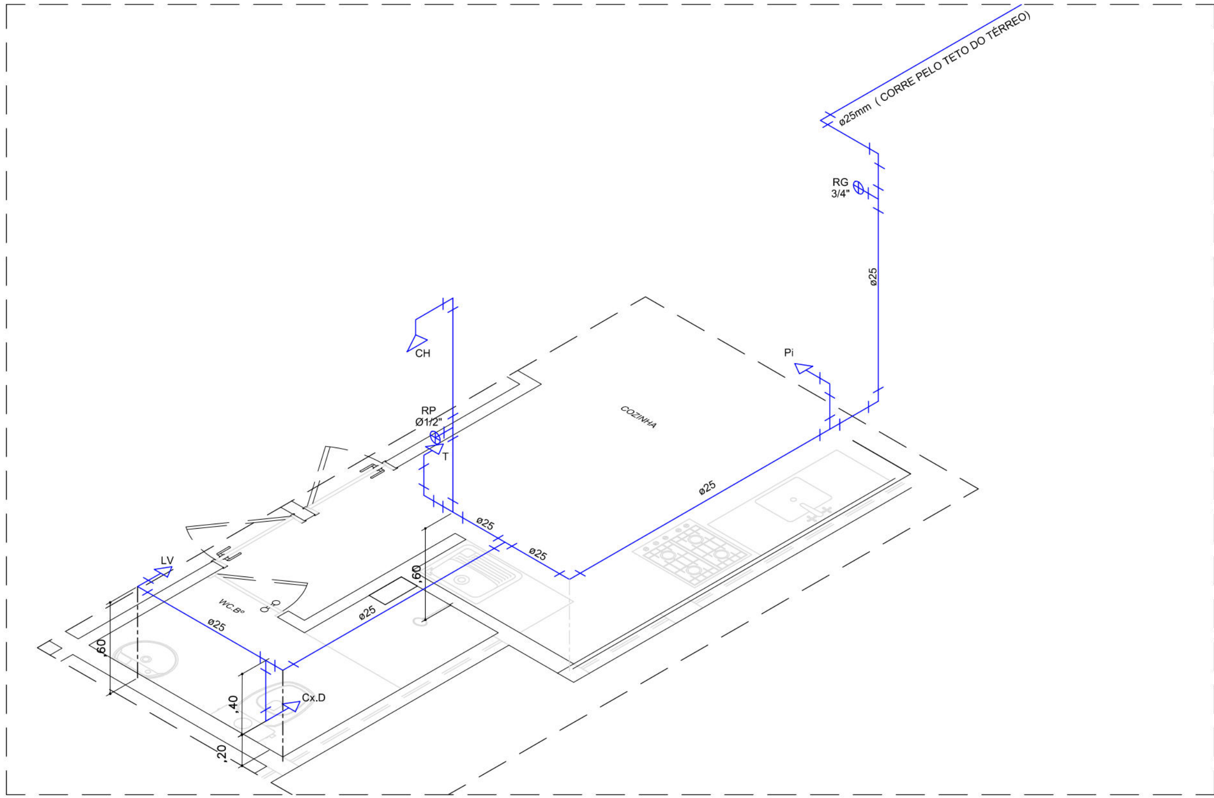
DETALHE 2 ( ISOMÉTRICO ) ESCALA: 1/25
