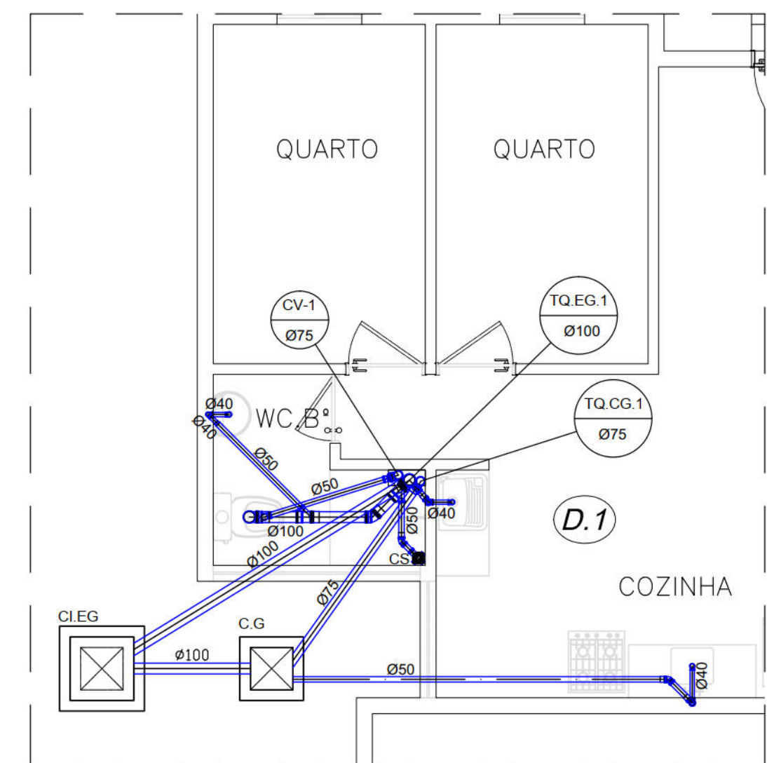
PLANTA BAIXA ESGOTO - TÉRREO ESCALA: 1/25
