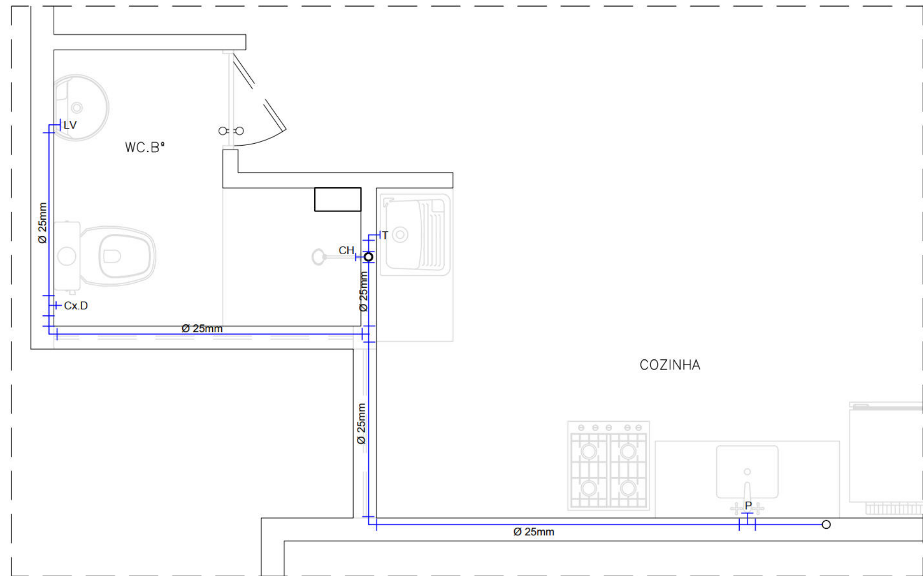
DETALHE 2 ( PLANTA BAIXA ) ESCALA: 1/50
