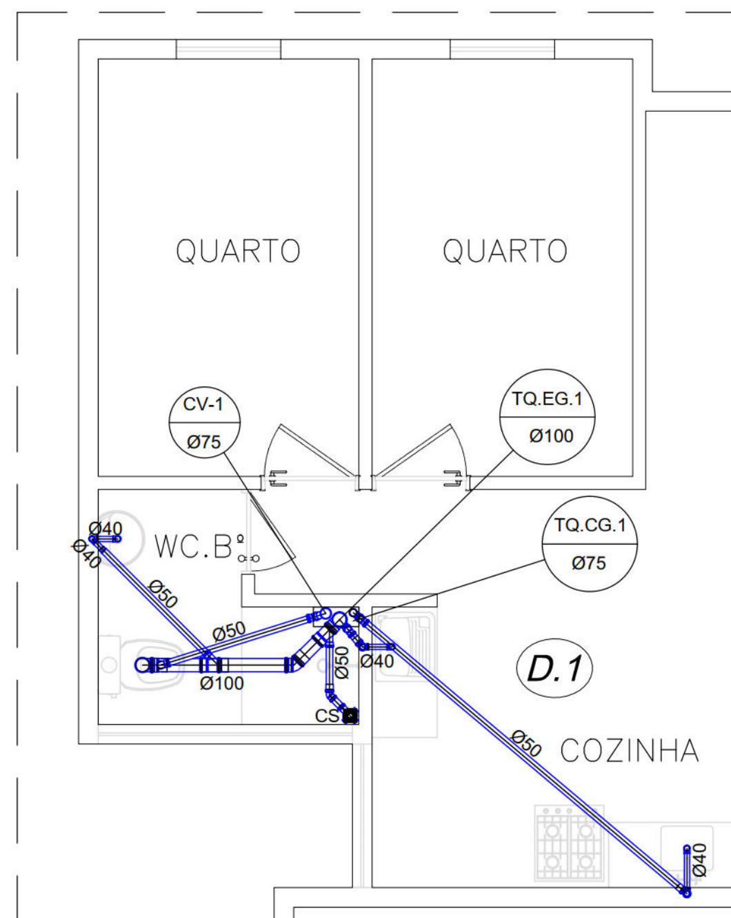
PLANTA BAIXA ESGOTO - 1º E 2º PAVIMENTO ESCALA: 1/25
