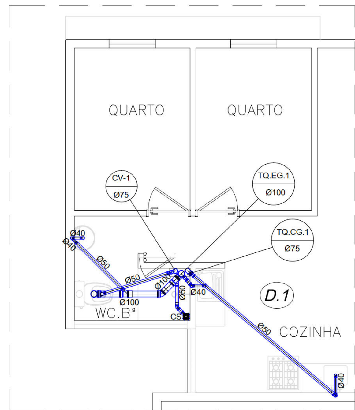
PLANTA BAIXA ESGOTO - 3º PAVIMENTO ESCALA: 1/25
