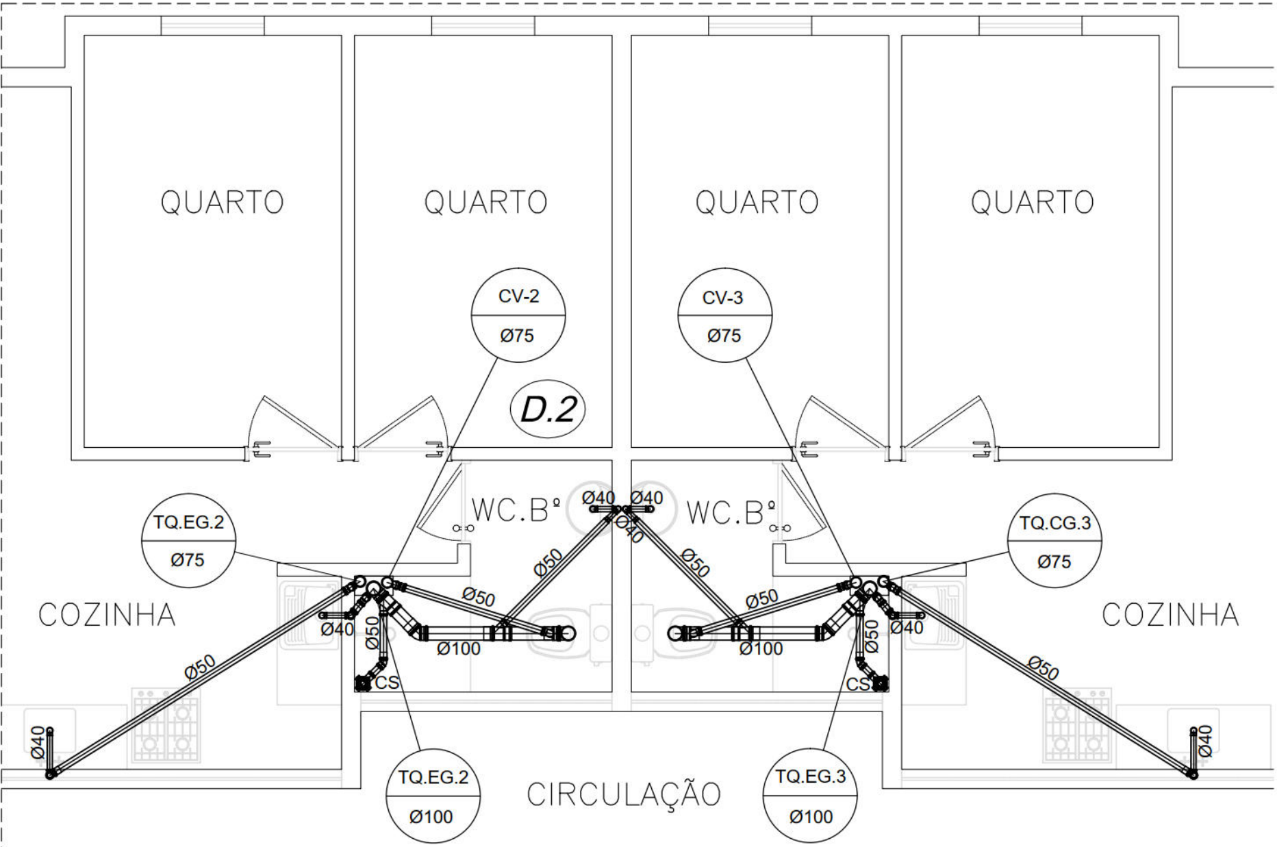
PLANTA BAIXA ESGOTO - 1º E 2º PAVIMENTO ESCALA: 1/25
