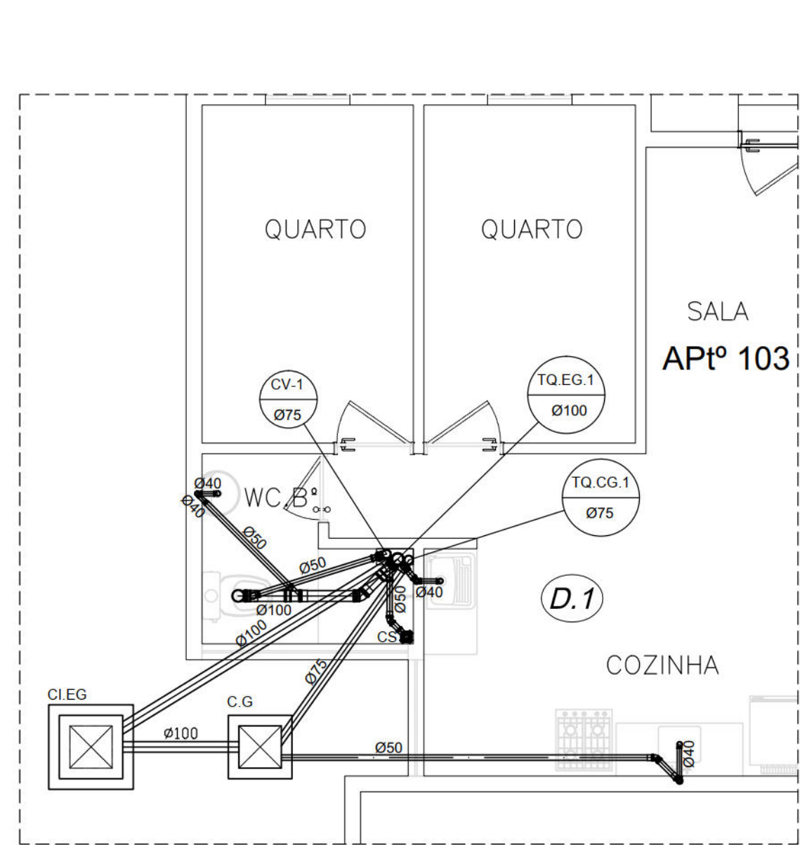
PLANTA BAIXA ESGOTO - TÉRREO ESCALA: 1/25
