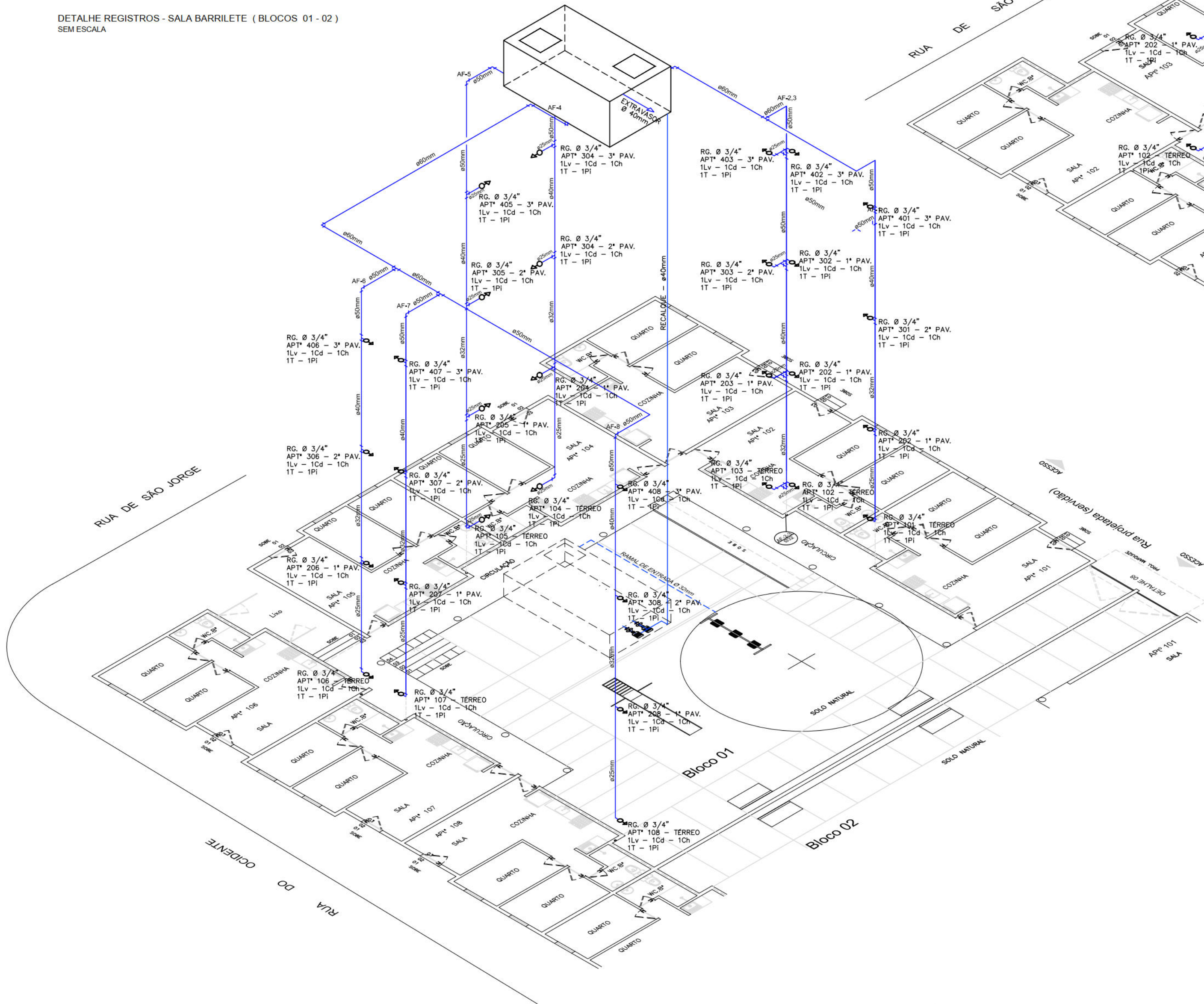
DETALHE ISOMÉTRICO - ÁGUA FRIA SEM ESCALA
