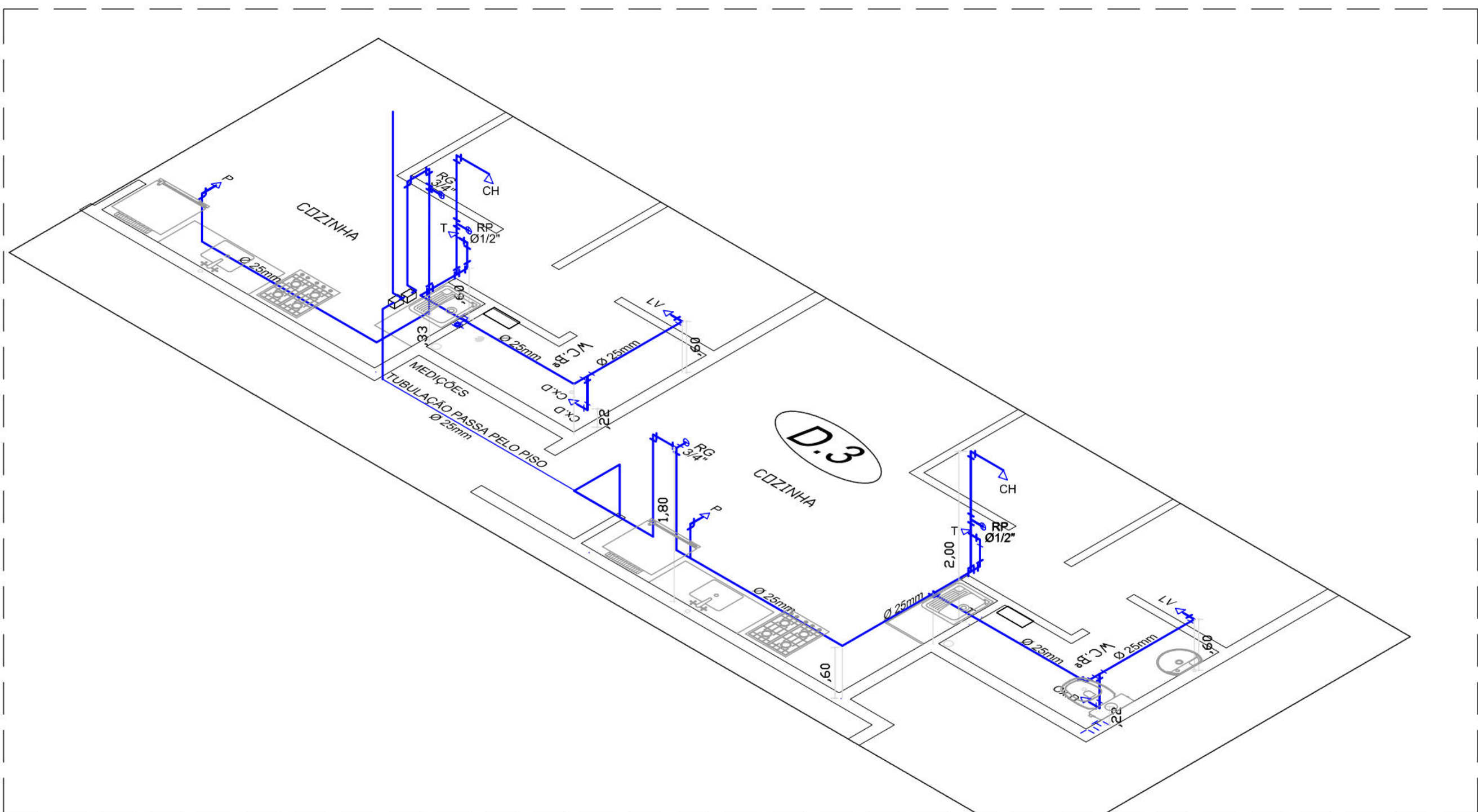
ISOMETRIA 3 ( PLANTA BAIXA - TÉRREO ) ESCALA: 1/50
