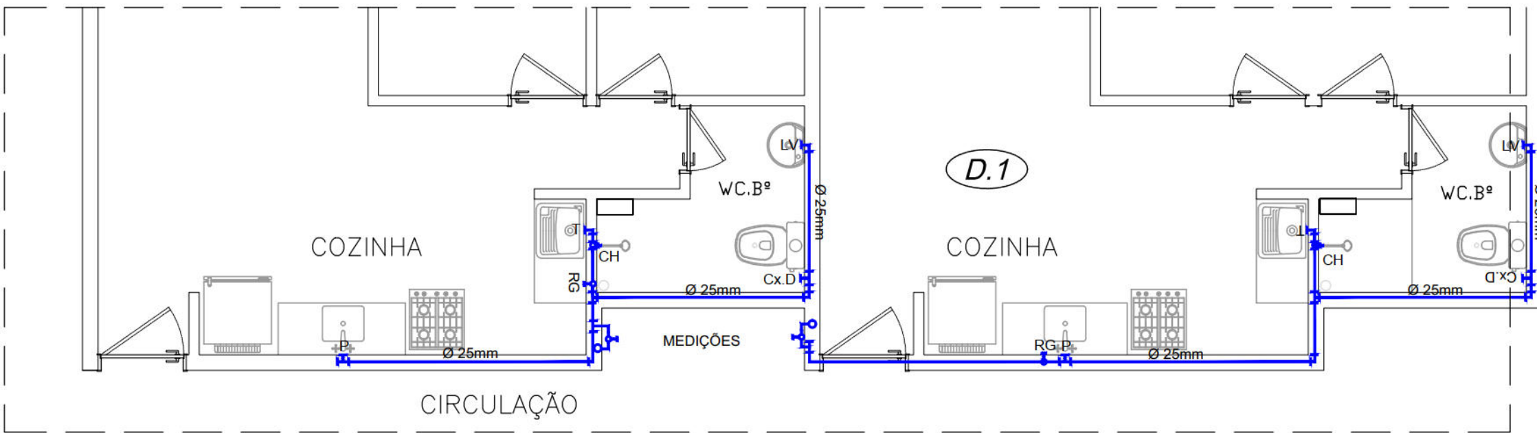
DETALHE 1 ( PLANTA BAIXA - TÉRREO ) ESCALA: 1/50
