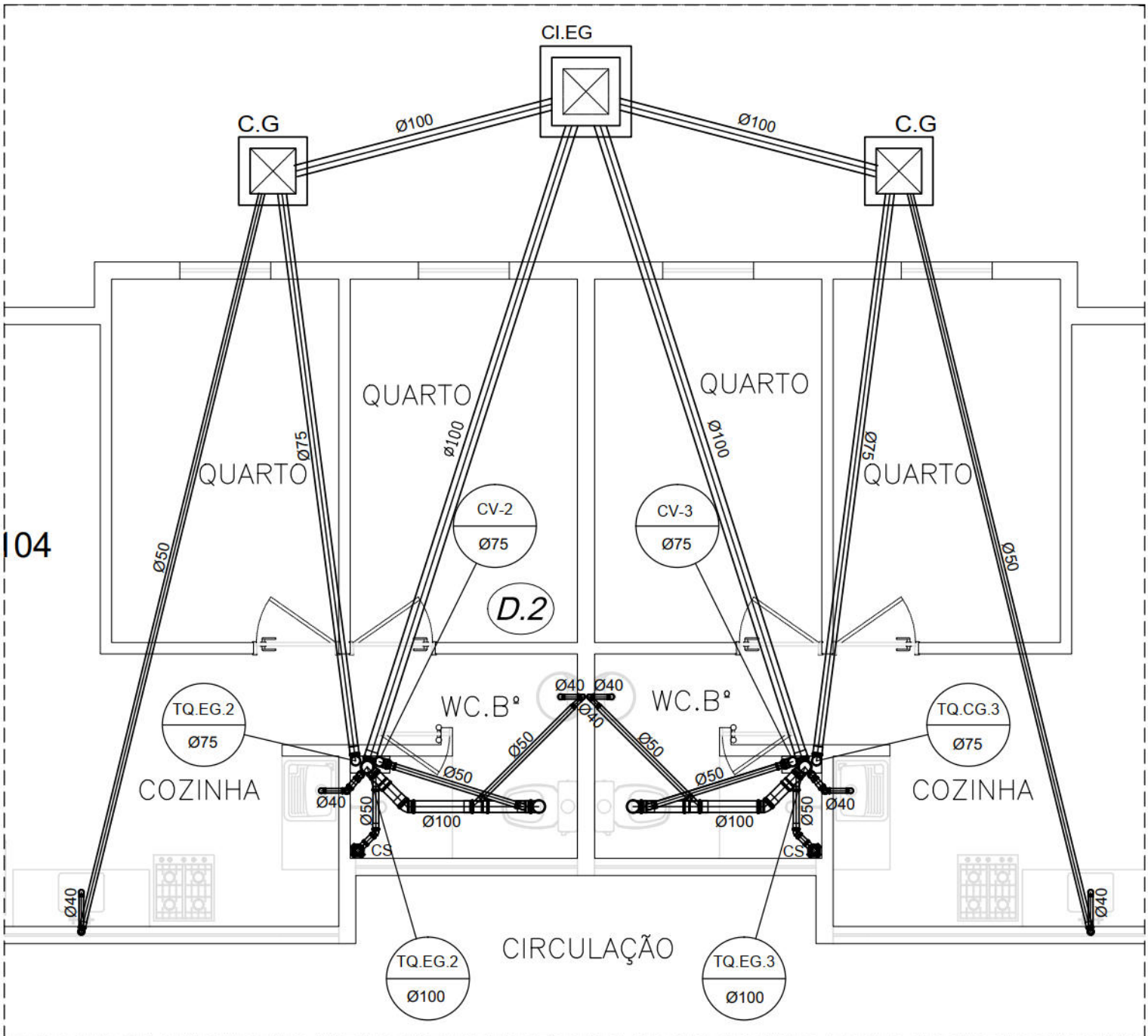
PLANTA BAIXA ESGOTO - TÉRREO ESCALA: 1/25
