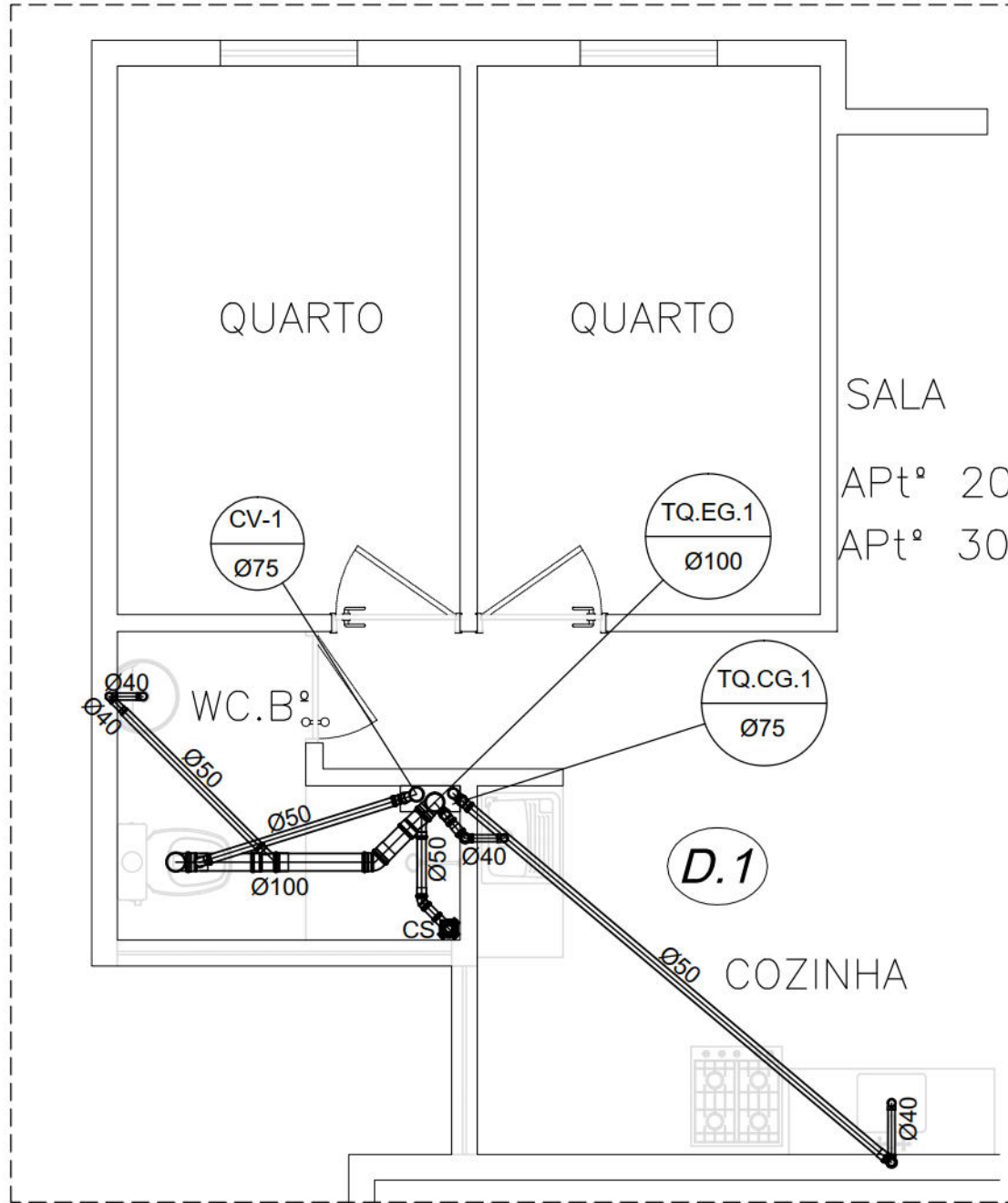
PLANTA BAIXA ESGOTO - 1º E 2º PAVIMENTO ESCALA: 1/25
