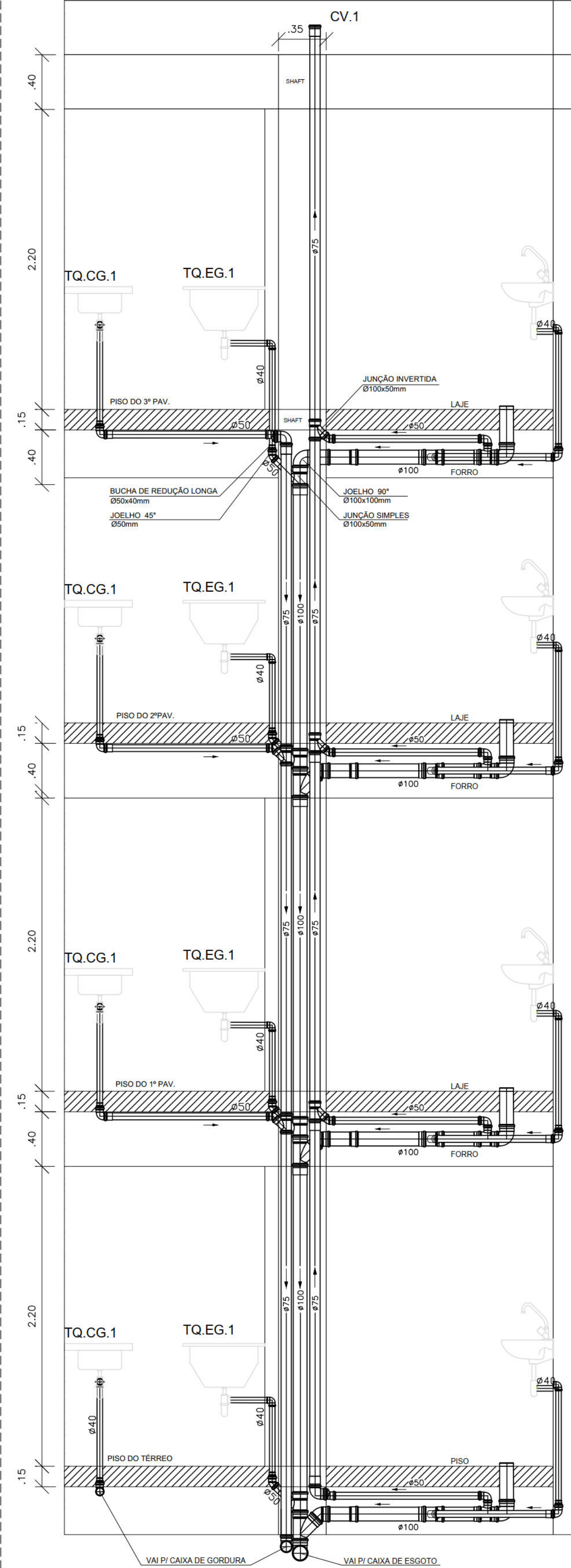
VISTA LATERAL SEM ESCALA
