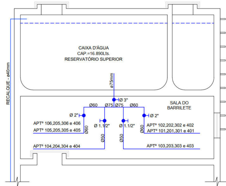
DETALHE REGISTROS - SALA BARRILETE ( BLOCO 03 ) SEM ESCALA
