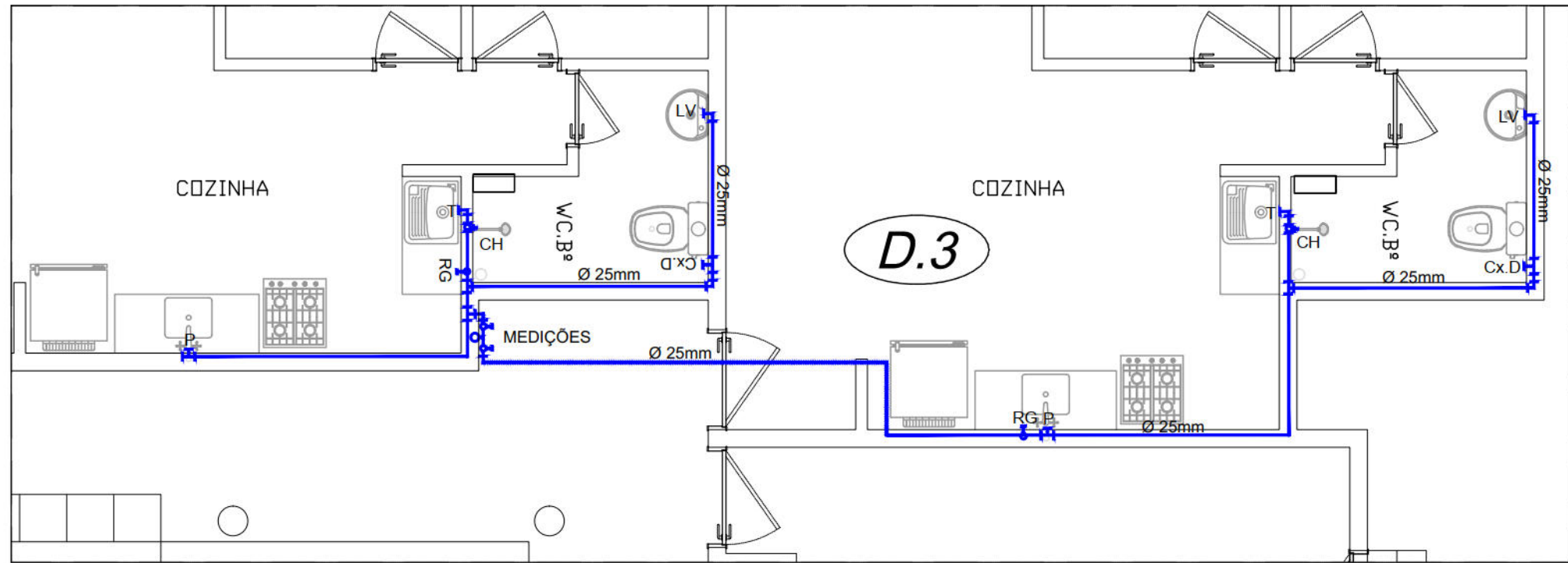
DETALHE 3 ( PLANTA BAIXA - TÉRREO ) ESCALA: 1/50
