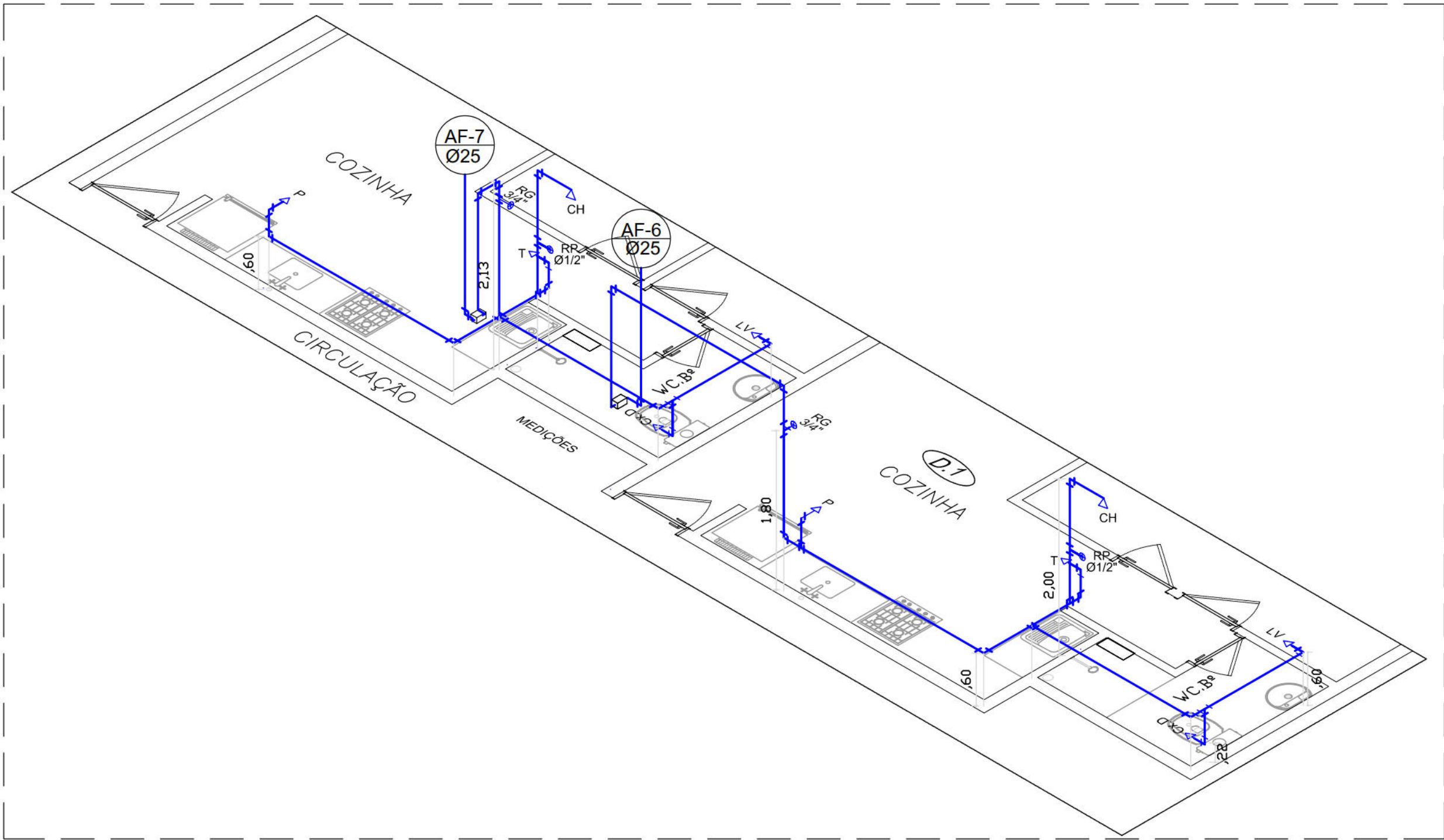
ISOMETRIA 1 ( PLANTA BAIXA - TÉRREO ) ESCALA: 1/50
