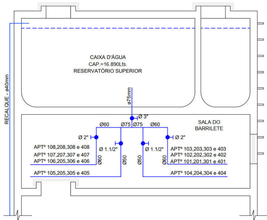
DETALHE REGISTROS - SALA BARRILETE ( BLOCOS 01 - 02 ) SEM ESCALA
