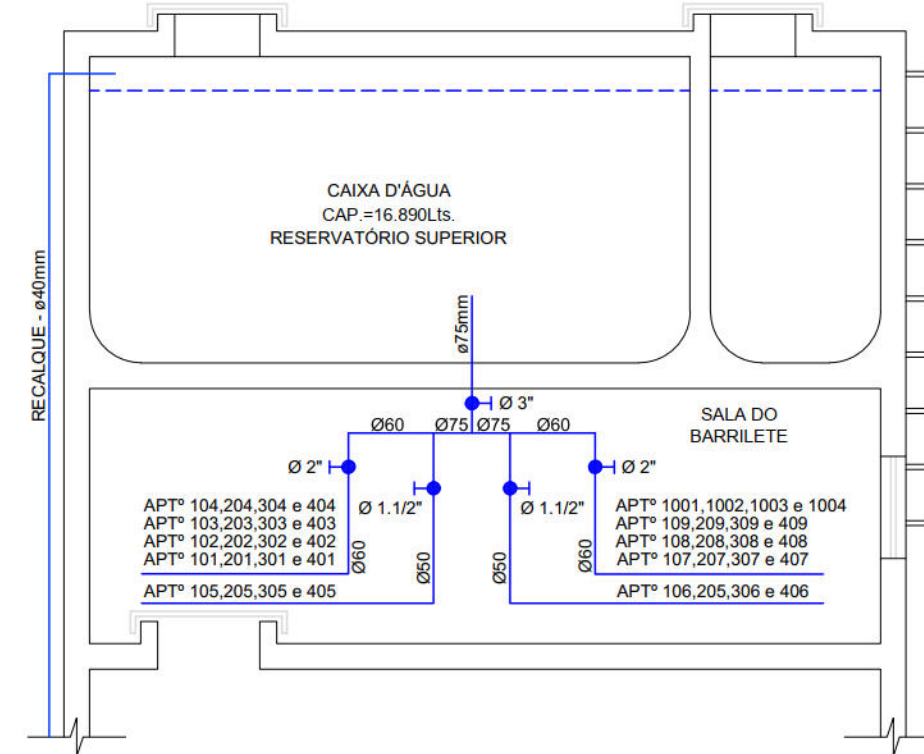
DETALHE REGISTROS - SALA BARRILETE ( BLOCO 04 ) SEM ESCALA
