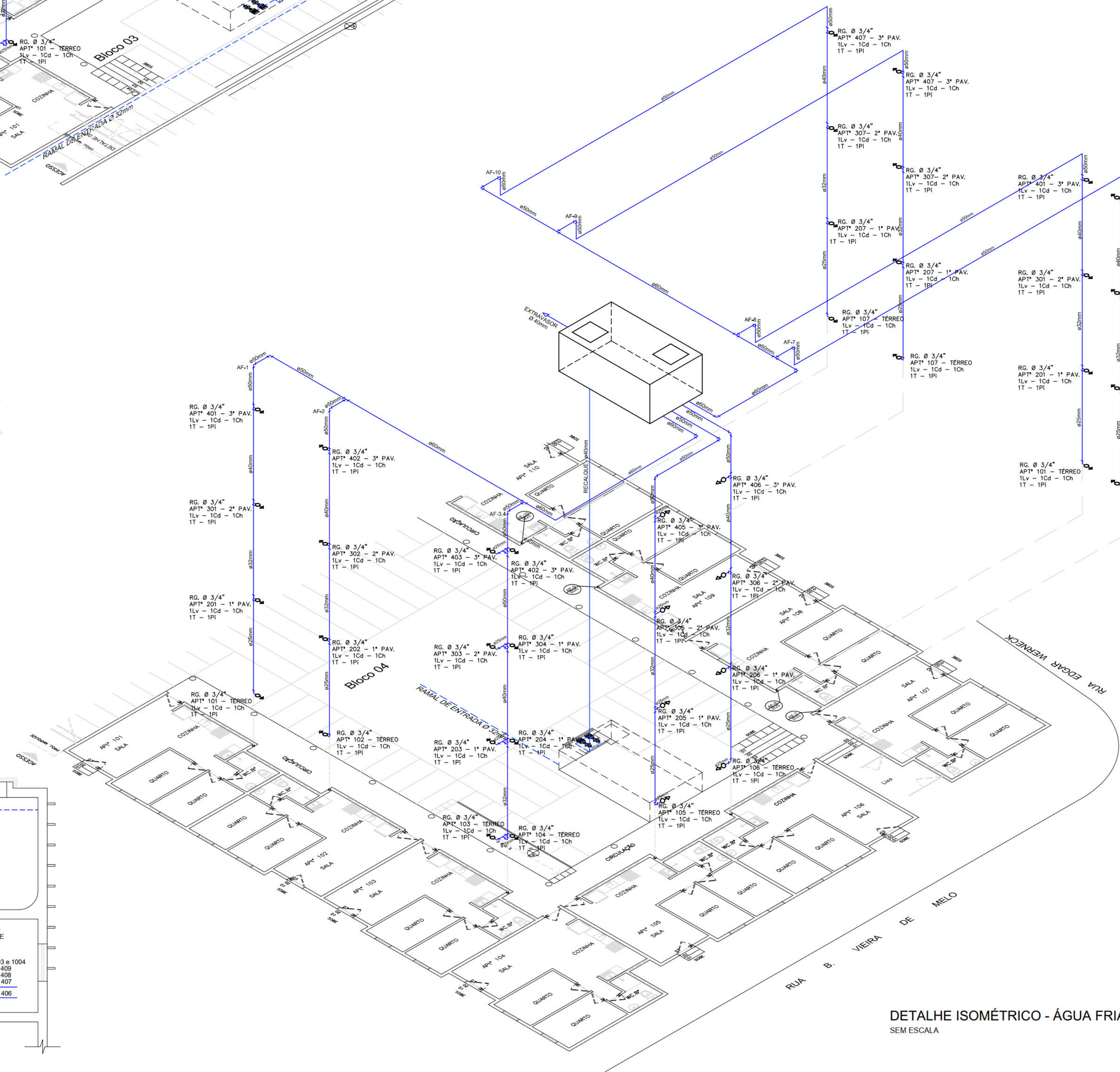
DETALHE ISOMÉTRICO - ÁGUA FRIA SEM ESCALA
