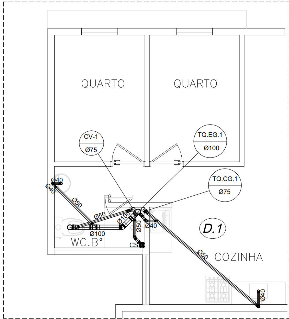
PLANTA BAIXA ESGOTO - 3º PAVIMENTO ESCALA: 1/25
