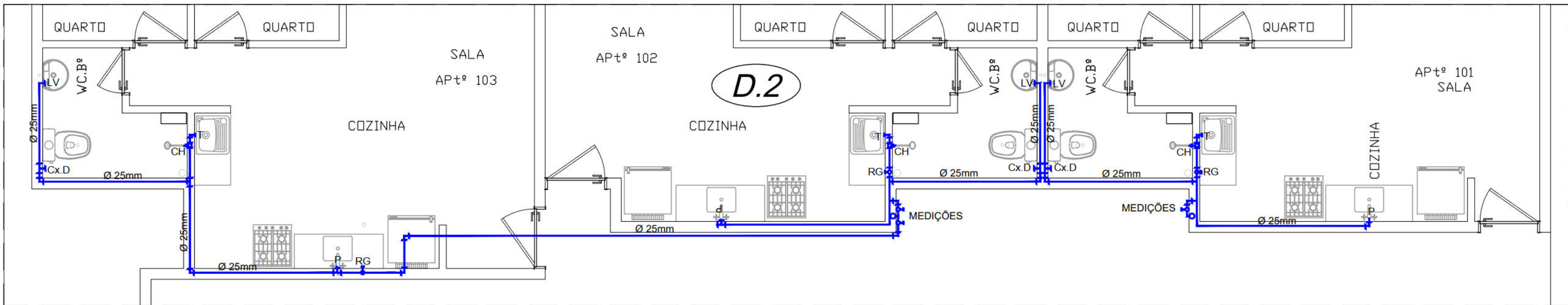
DETALHE 2 ( PLANTA BAIXA - TÉRREO ) ESCALA: 1/50
