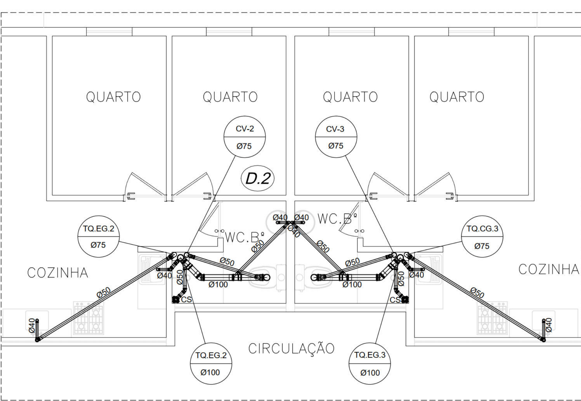
PLANTA BAIXA ESGOTO - 3º PAVIMENTO ESCALA: 1/25
