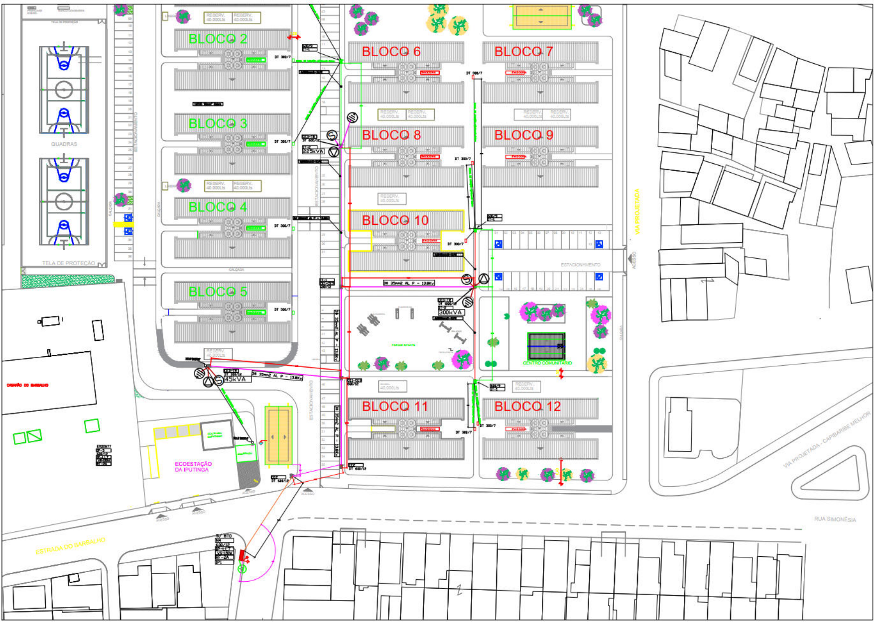
PLANTA DE SITUAÇÃO ESC 1:1000
