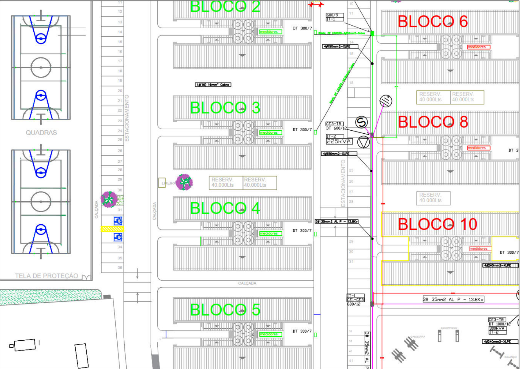
PLANTA DE LOCAÇÃO ESC 1:500
