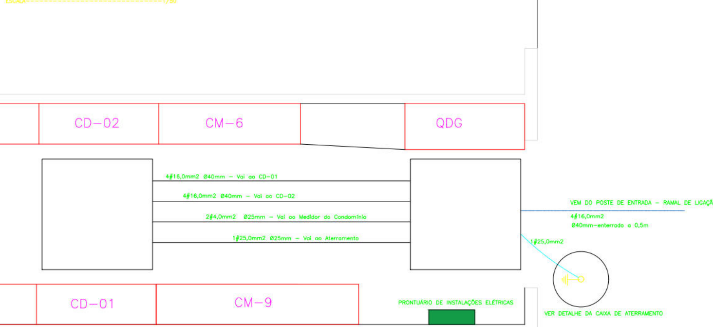
PLANTA DOS MEDIDORES
