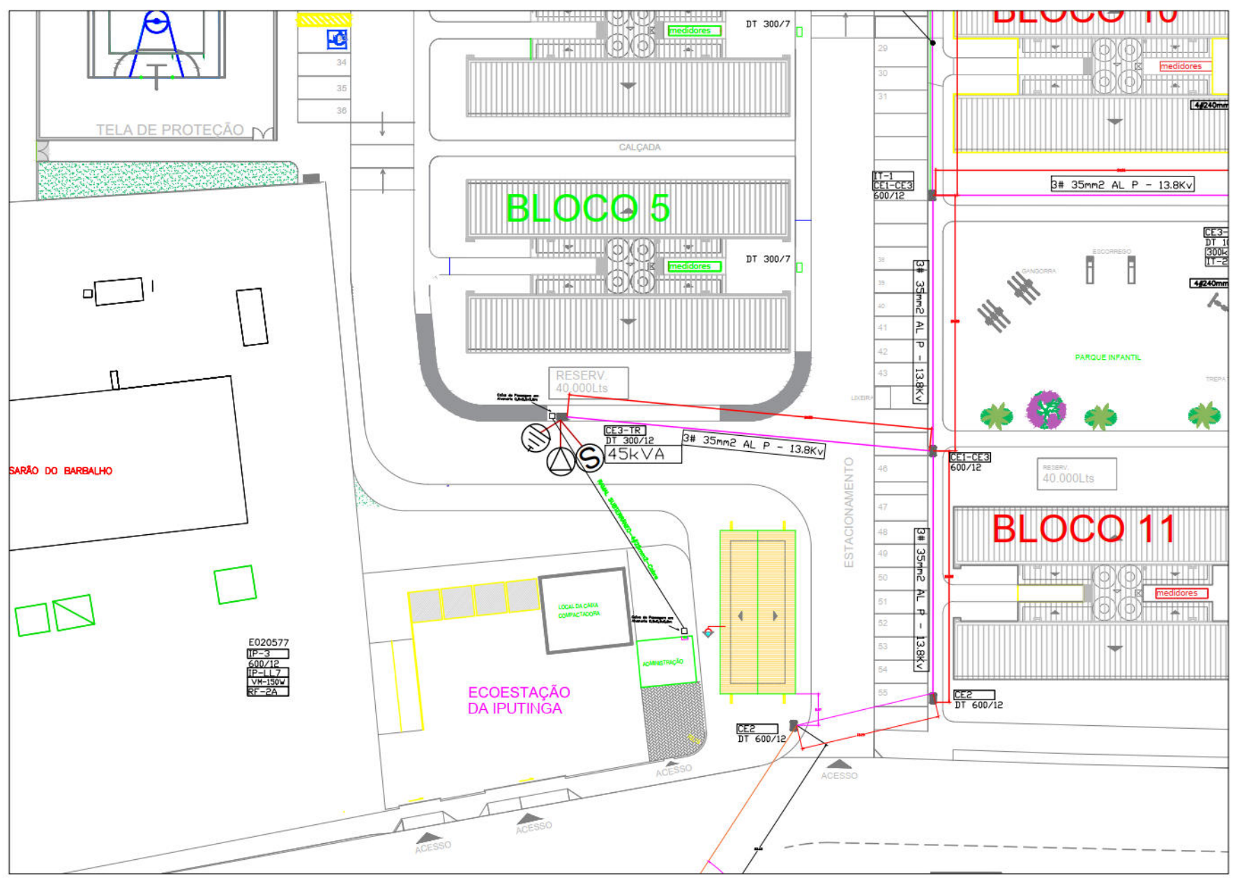
PLANTA DE LOCAÇÃO ESC 1:500
