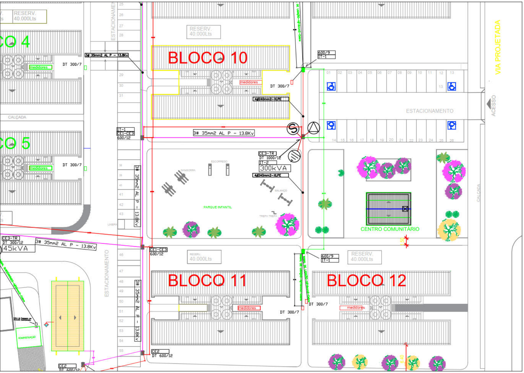
PLANTA DE LOCAÇÃO ESC 1:500
