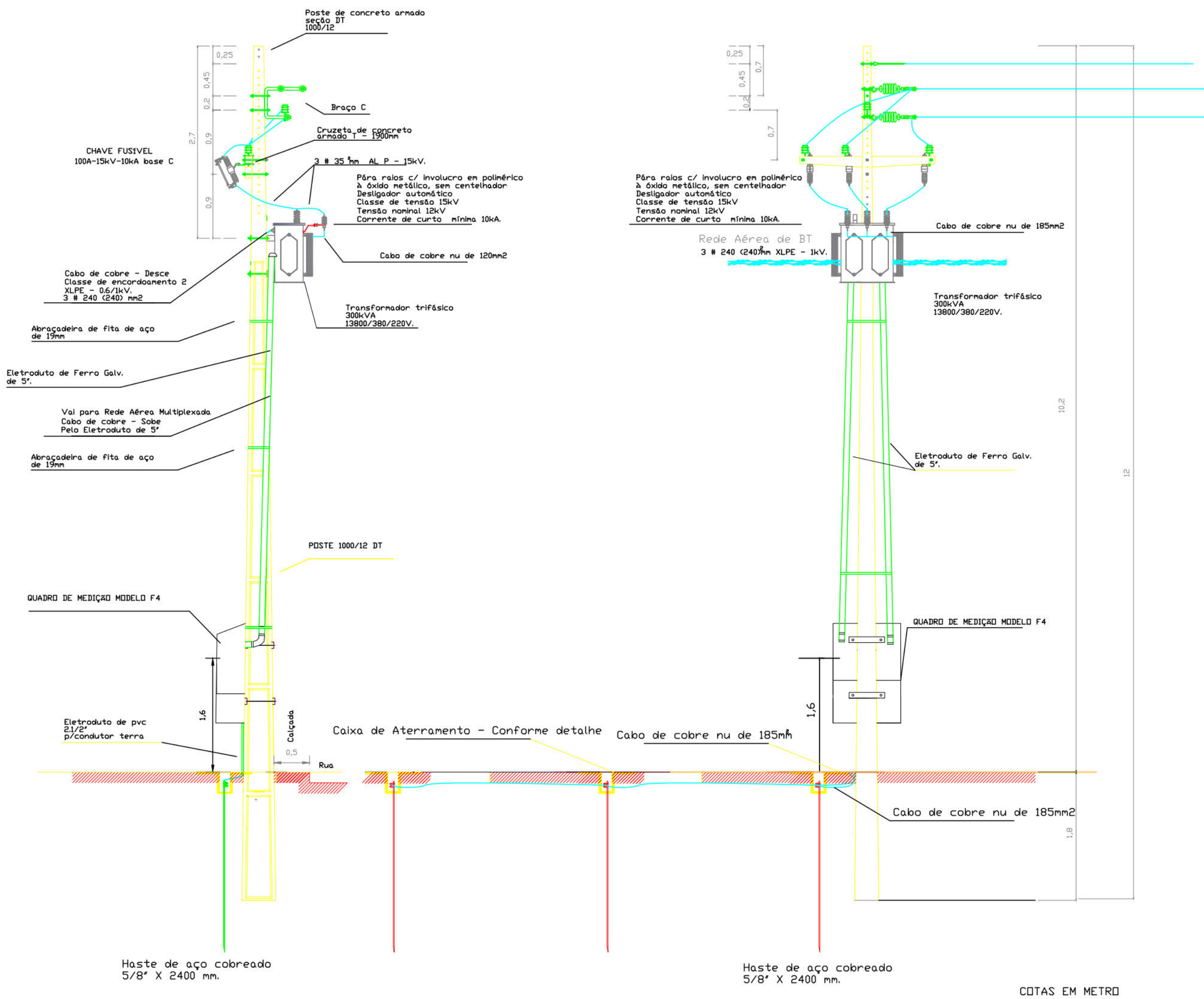
VISTA LATERAL - ESC 1/50
