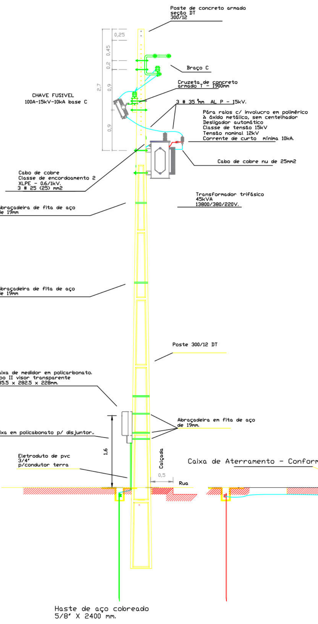
VISTA LATERAL - ESC 1/50
