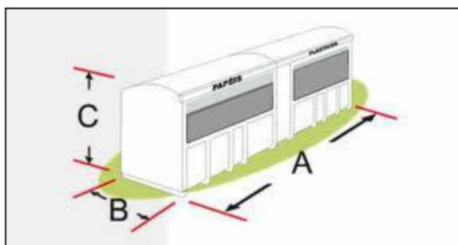
Figura 2 – Modelo de baias utilizadas para o armazenamento final de alguns resíduos no canteiro de obras
