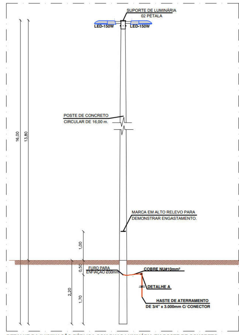
DETALHE DE ILUMINAÇÃO PÚBLICA COM DUAS LUMINÁRIAS EM POSTE DE CONCRETO DE DEZESSEIS METROS. ESCALA: 1/50
