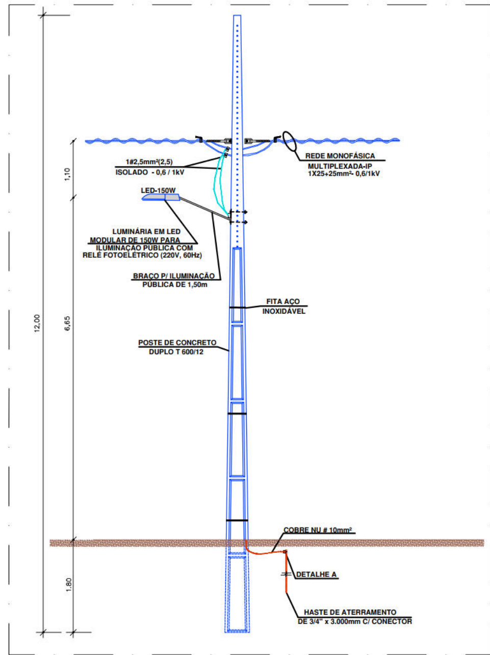
DETALHE DE ILUMINAÇÃO PÚBLICA PARA UMA LUMINÁRIA EM POSTE DE CONCRETO DE 12 METROS. ESCALA: 1/50
