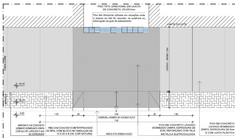
Figura 3 - Rampa padrão para o acesso de veículos
