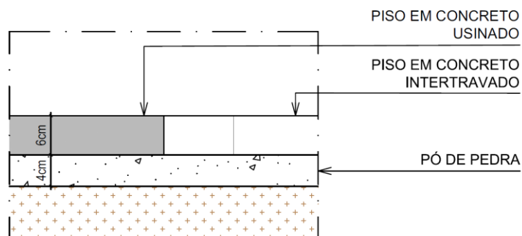
Figura 8 - Seção de Pavimentação Genérica
