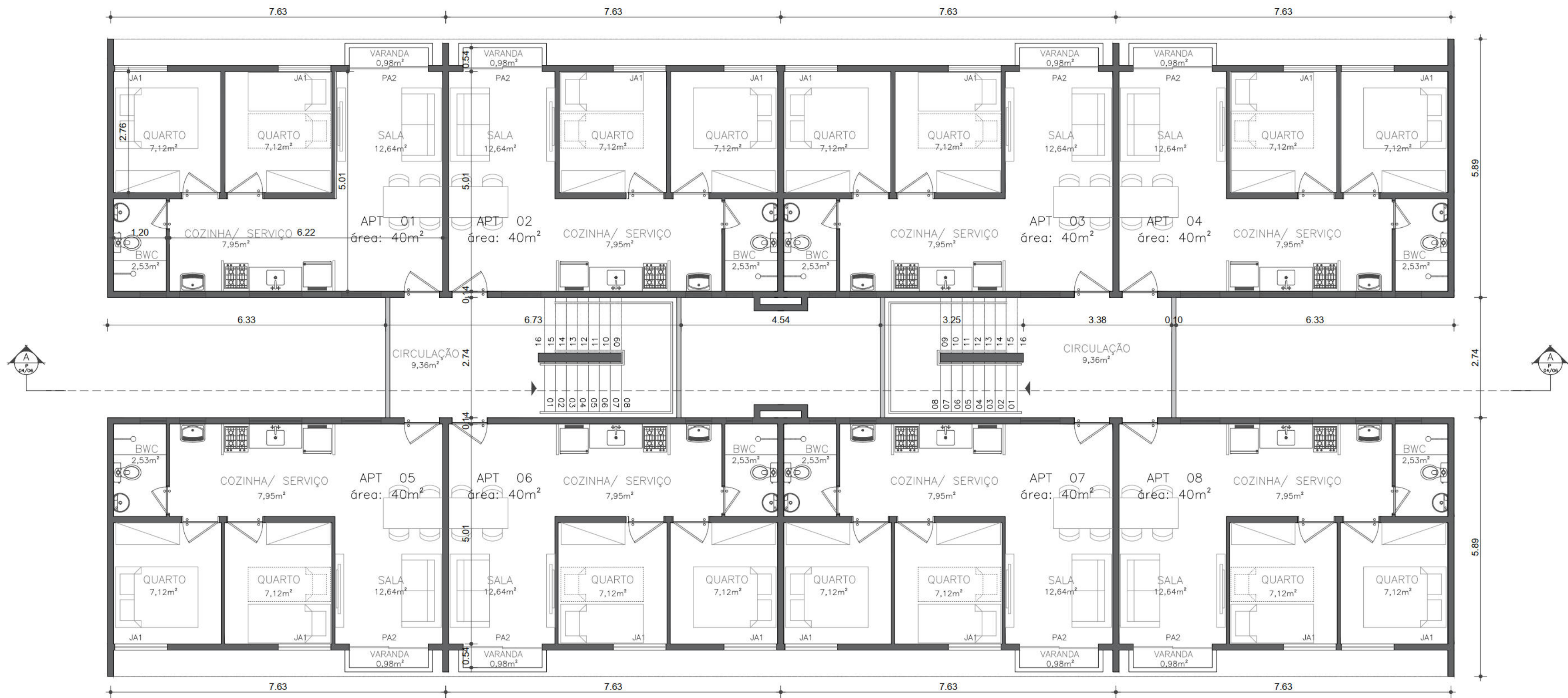
PLANTA BAIXA PAVIMENTO TIPO - BLOCO 1 ESC: 1/75
