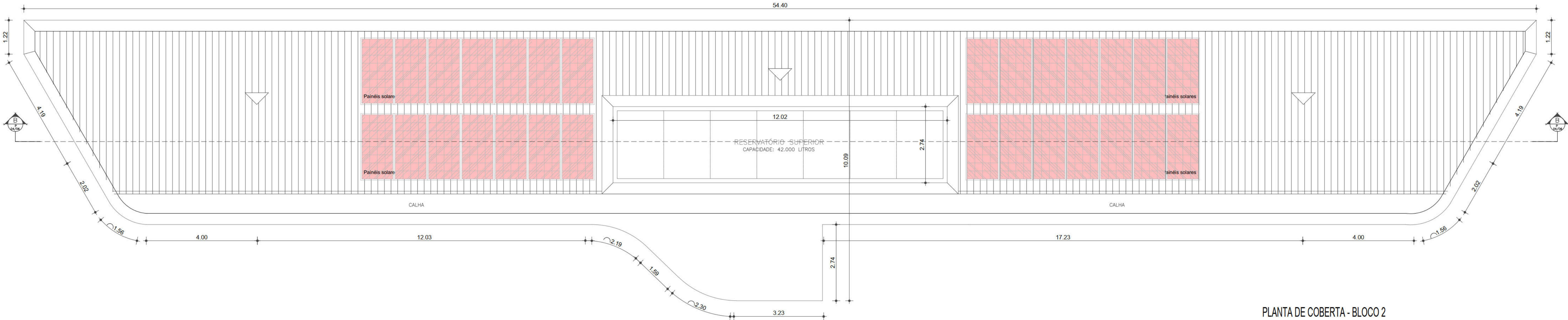
PLANTA DE COBERTA - BLOCO 2 ESC: 1/75
