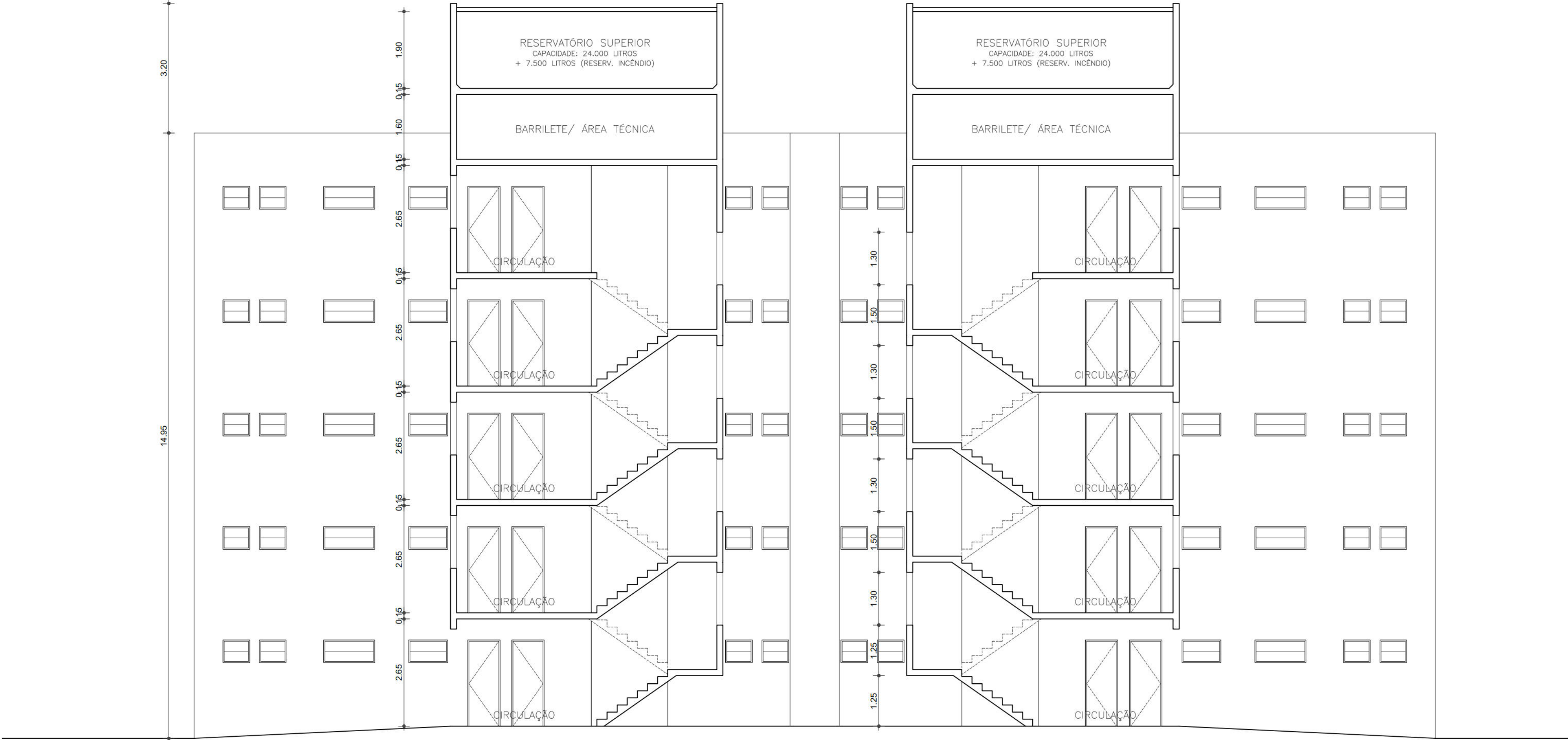
CORTE AA - BLOCO 1 ESC: 1/75
