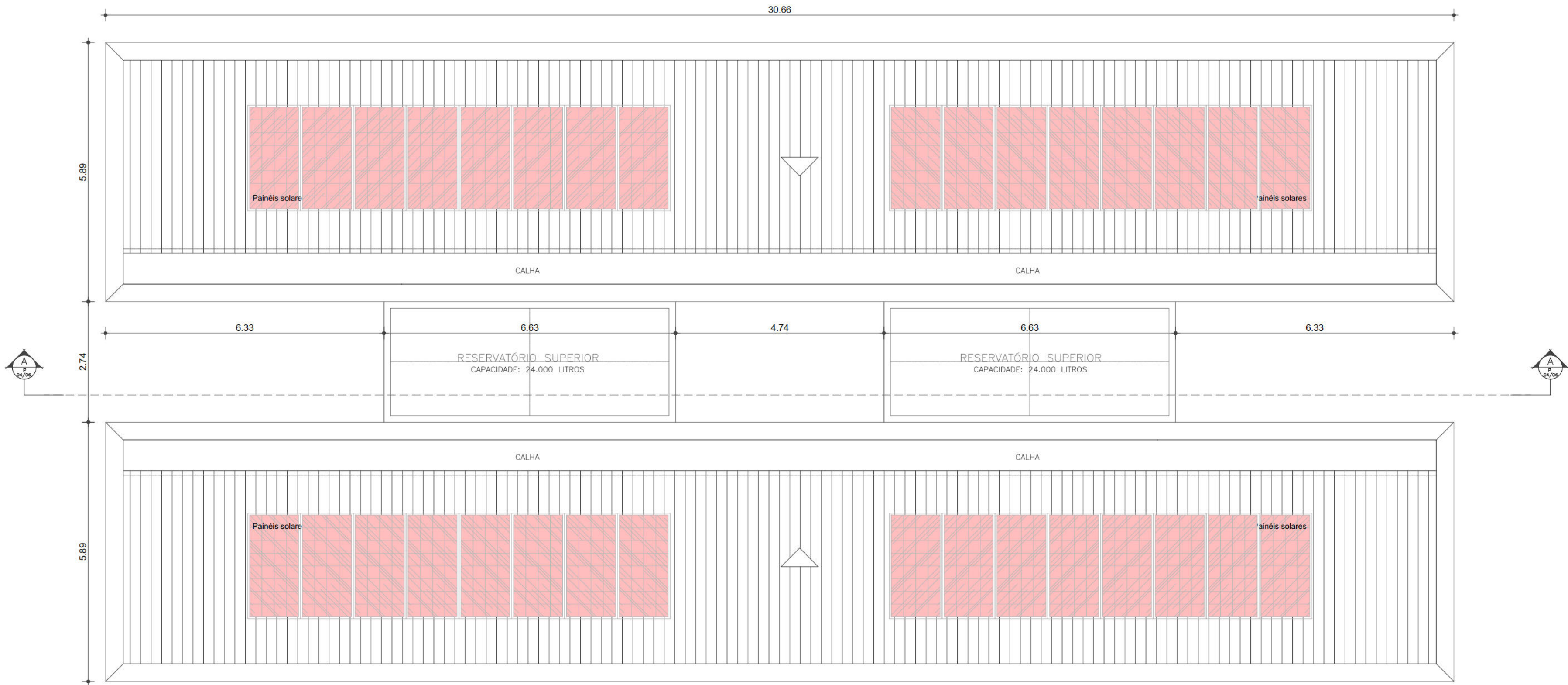
PLANTA DE COBERTA - BLOCO 1 ESC: 1/75
