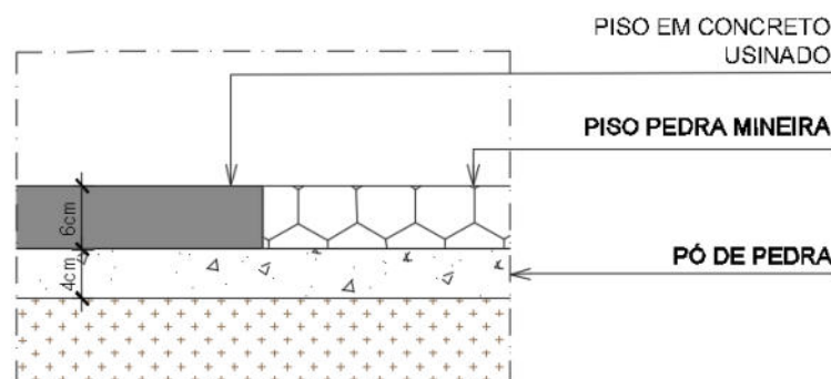
Figura 11 - Seção Tipo de Pavimentação
