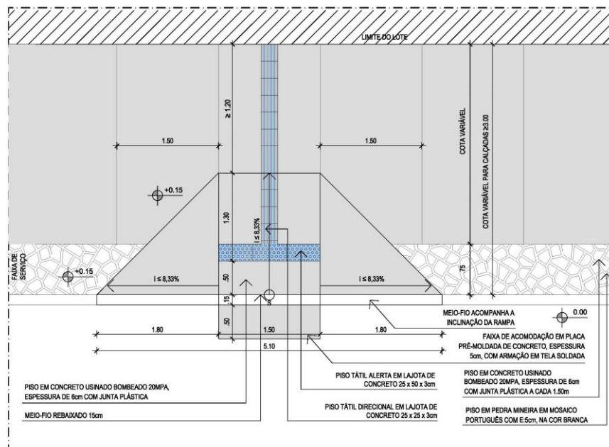
Figura 6 - Rampa para o acesso de pedestres - TIPO A
