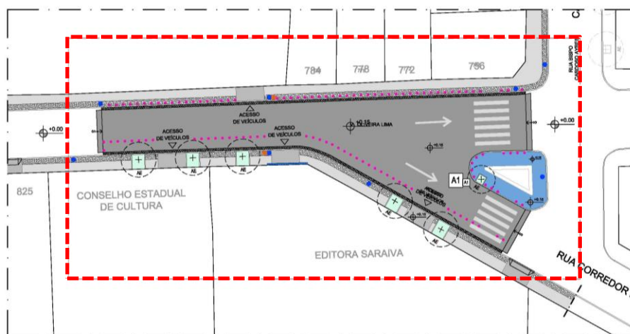
Figura 9 - Trecho Sem Desnível Entre Passeio e Via
