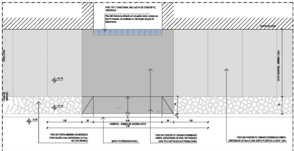
Figura 8 - Rampa padrão para o acesso de veículos
