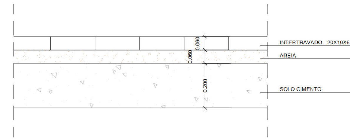
DETALHE - PISO ESCALA: 1:10
