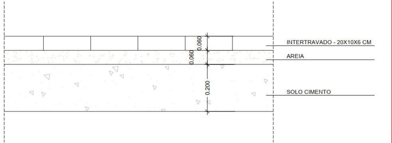
DETALHE - PISO ESCALA 1/10
