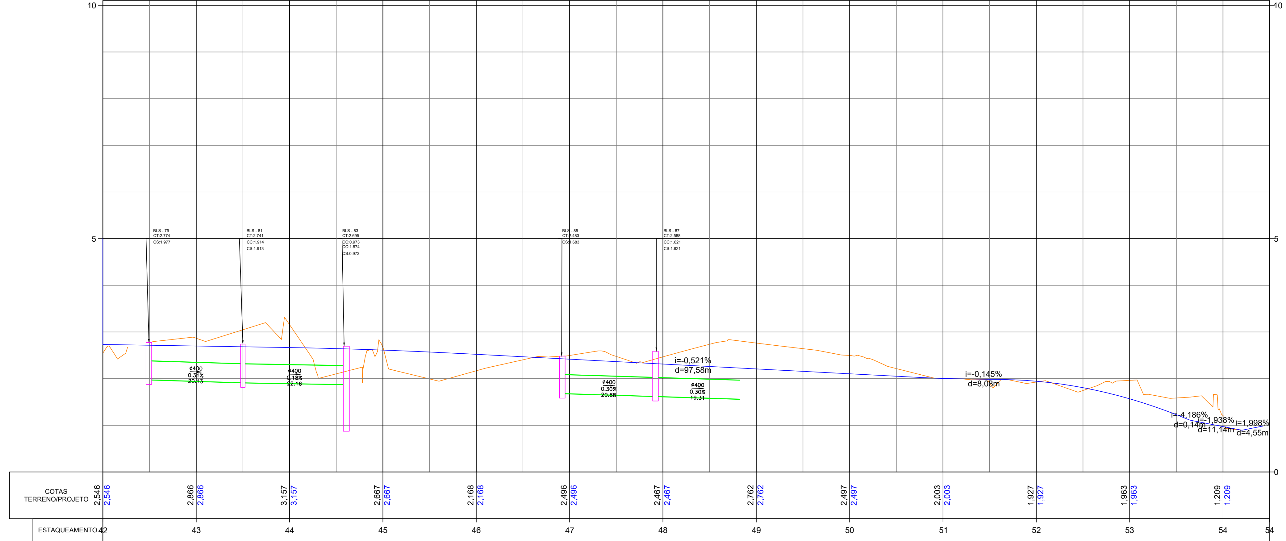
PERFIL ALINHAMENTO - ROTA ALTERNATIVA - LADO ESQUERDO
