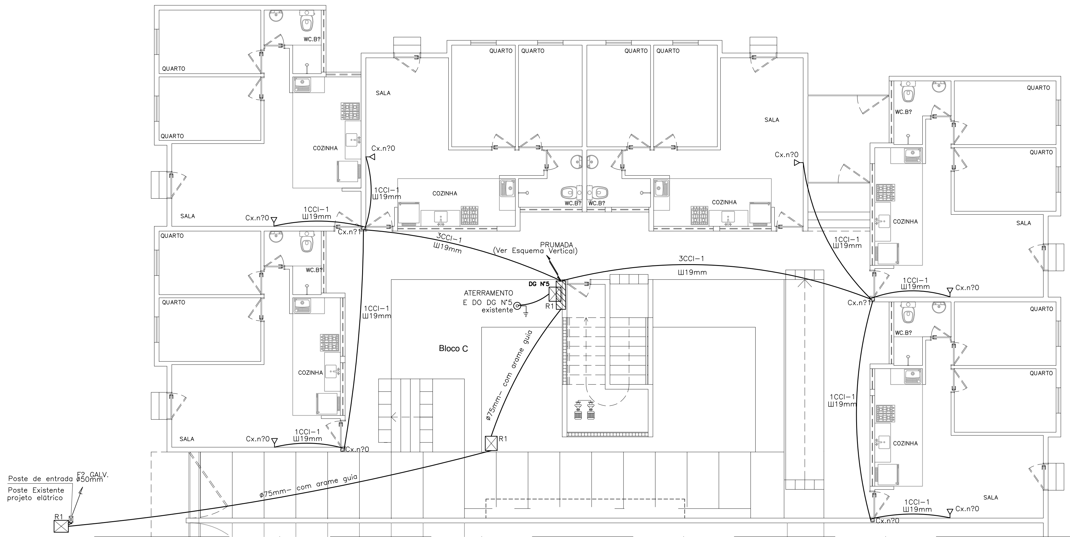
PLANTA BAIXA TIPO-REO-BLOCO C - QUADRA 55 ESCALA 1/75
