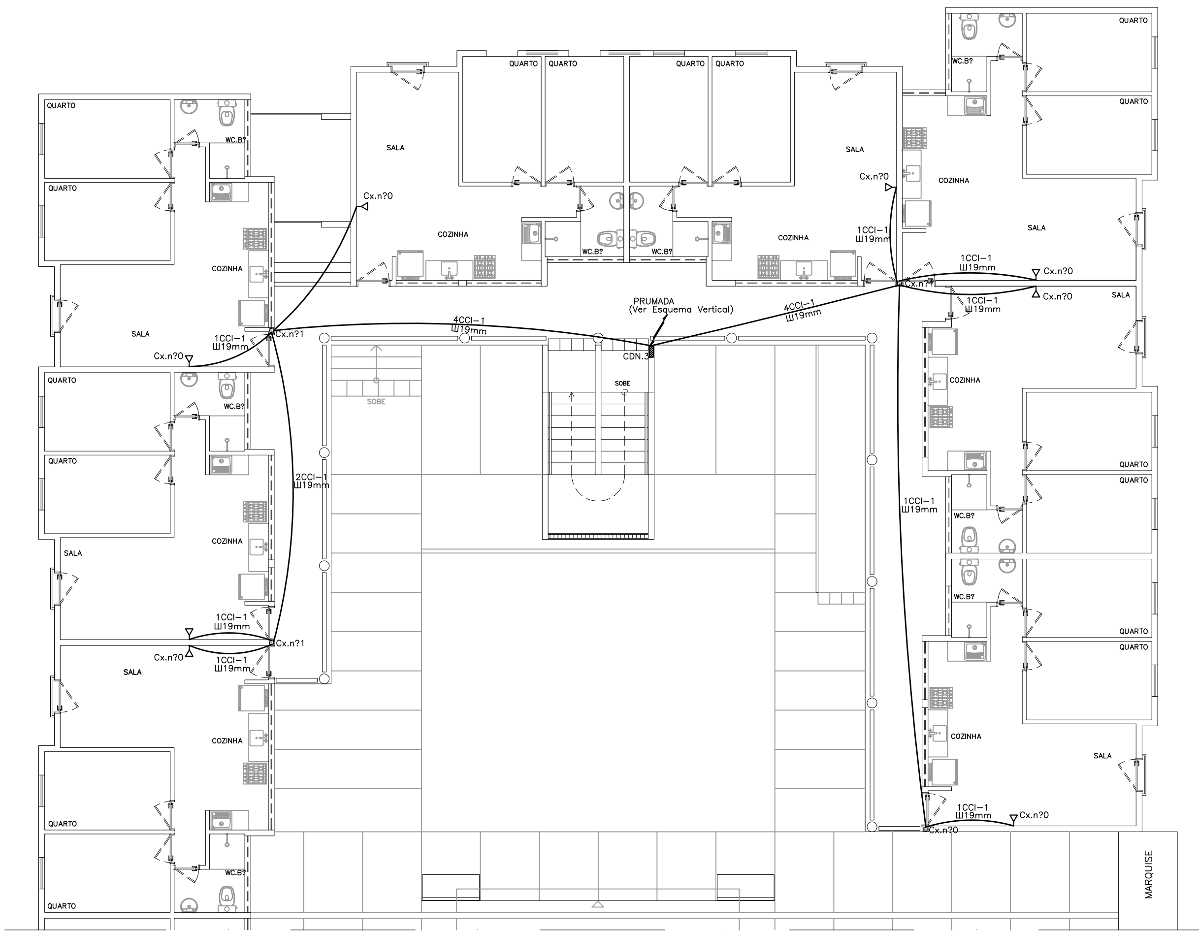
PLANTA BAIXA TIPO-BLOCO A - QUADRA 55 ESCALA 1/75
