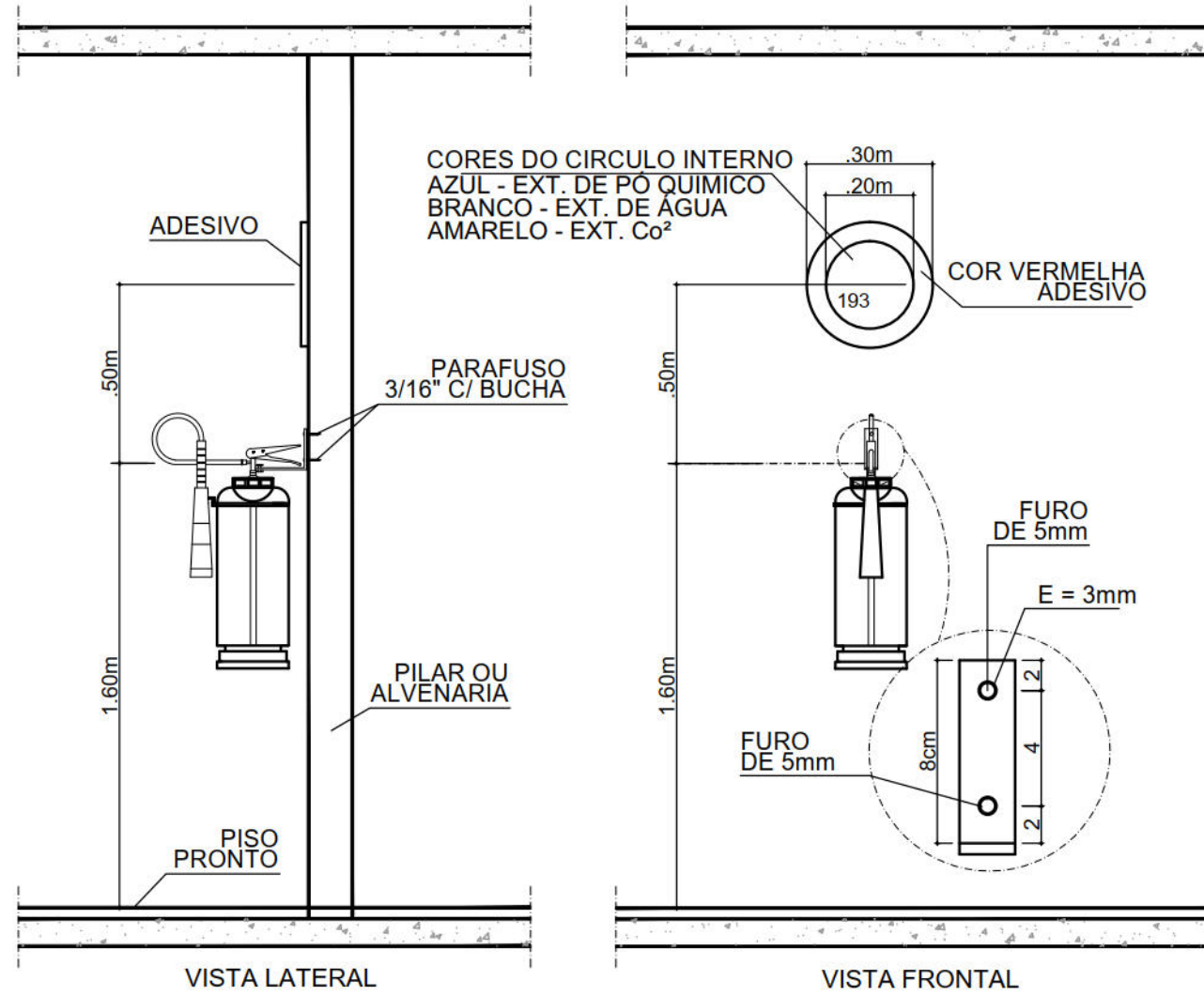
DETALHE FIXAÇÃO EXTINTOR S/ ESCALA
