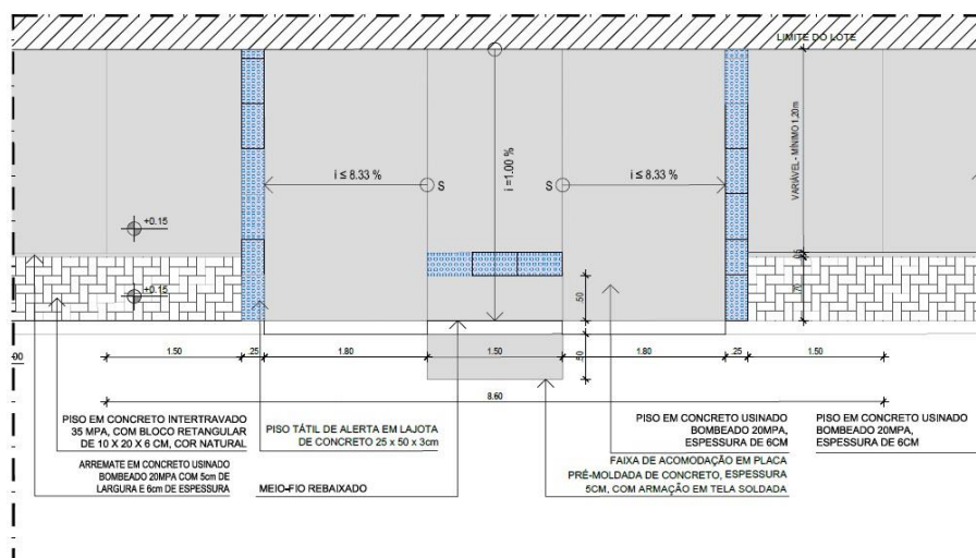
Figura 3 - Rampa para o acesso de pedestres - TIPO B
