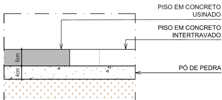
Figura 12 - Seção Tipo de Pavimentação
