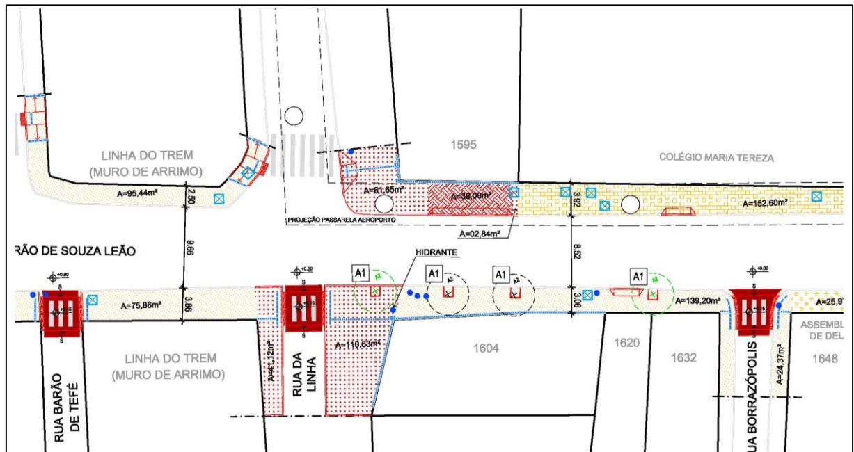
Figura 16 – Trecho de Implantação de Calçada
