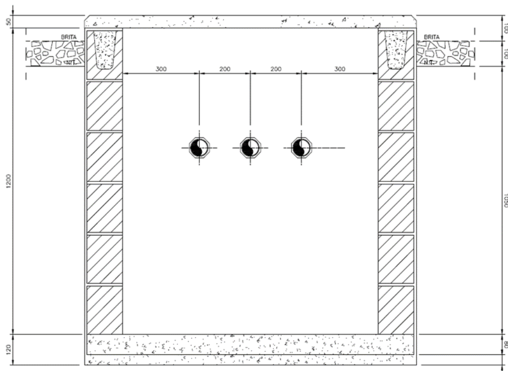
Figura 17 - Alternativa 01 - embutimento completo, corte A
