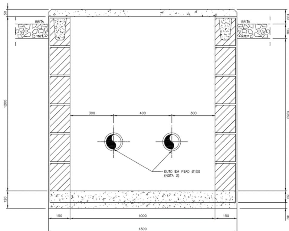
Figura 18 - Alternativa 01 - embutimento completo, corte B
