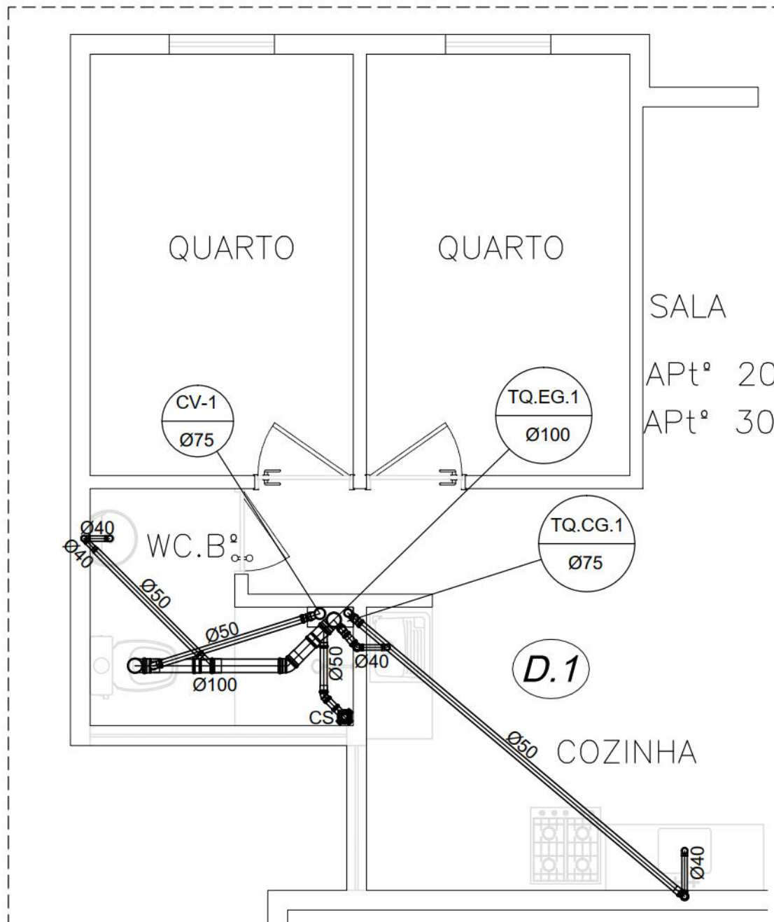
PLANTA BAIXA ESGOTO - 1º E 2º PAVIMENTO ESCALA: 1/25
