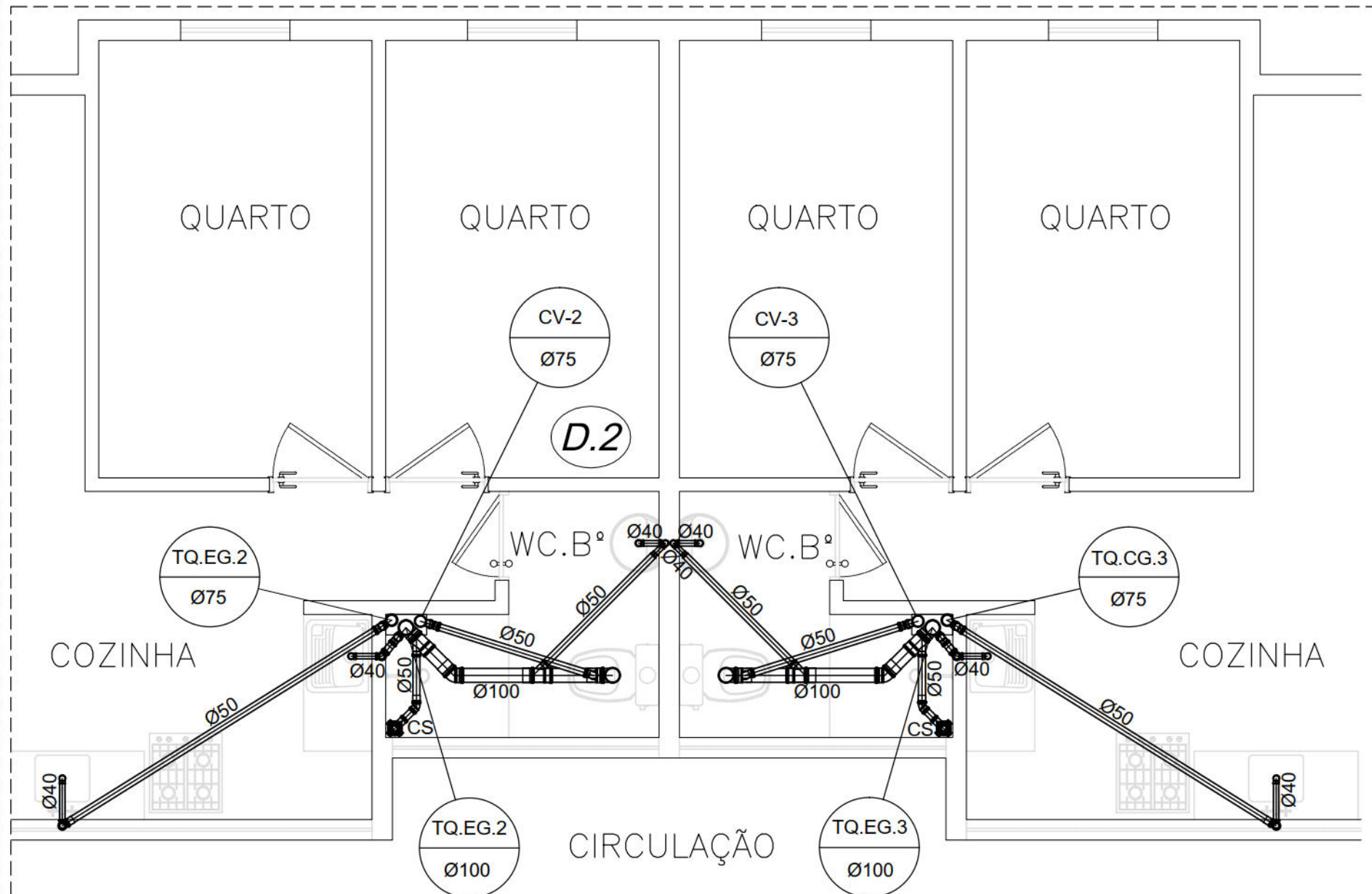
PLANTA BAIXA ESGOTO - 1º E 2º PAVIMENTO ESCALA: 1/25
