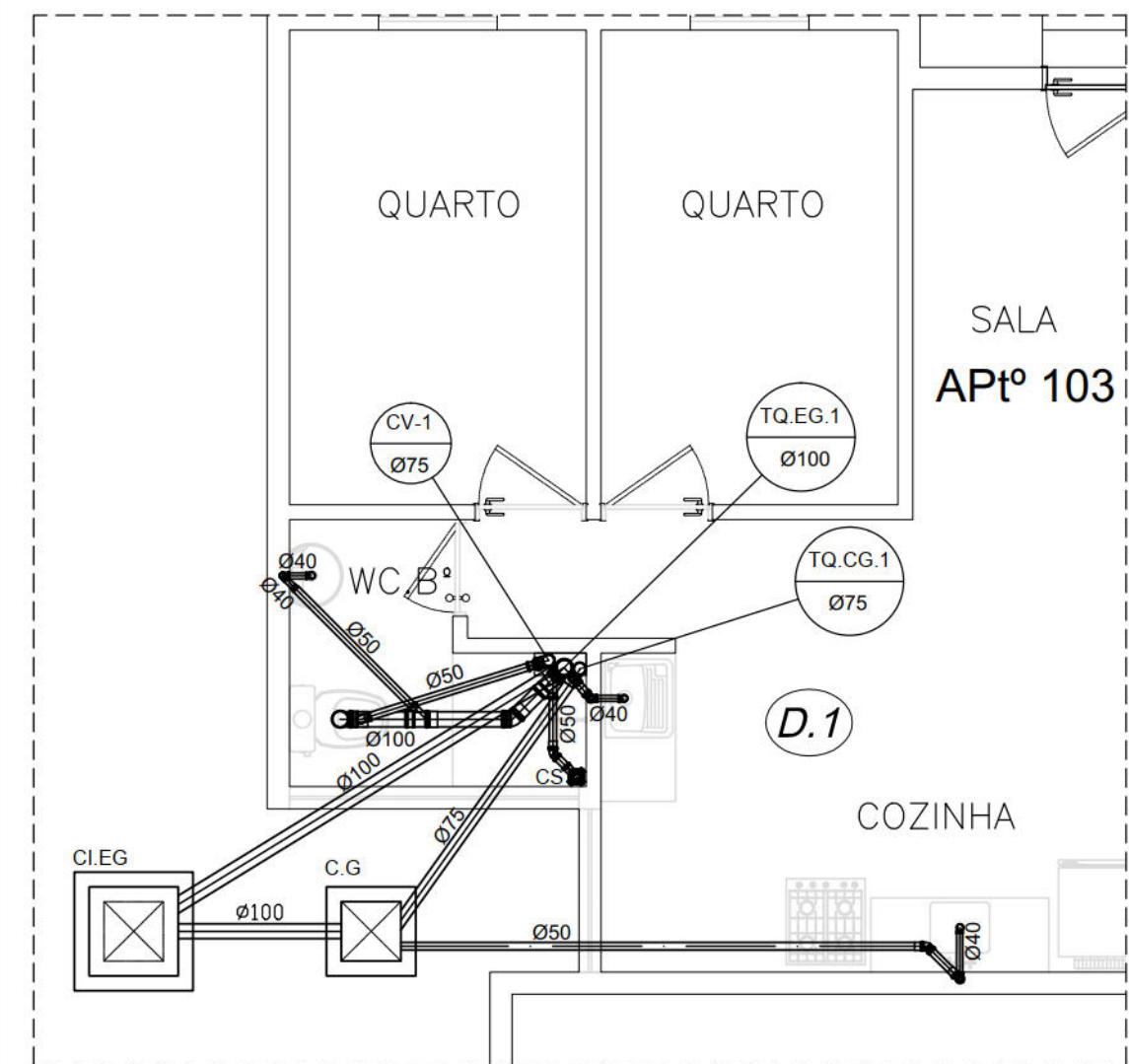
PLANTA BAIXA ESGOTO - TÉRREO ESCALA: 1/25
