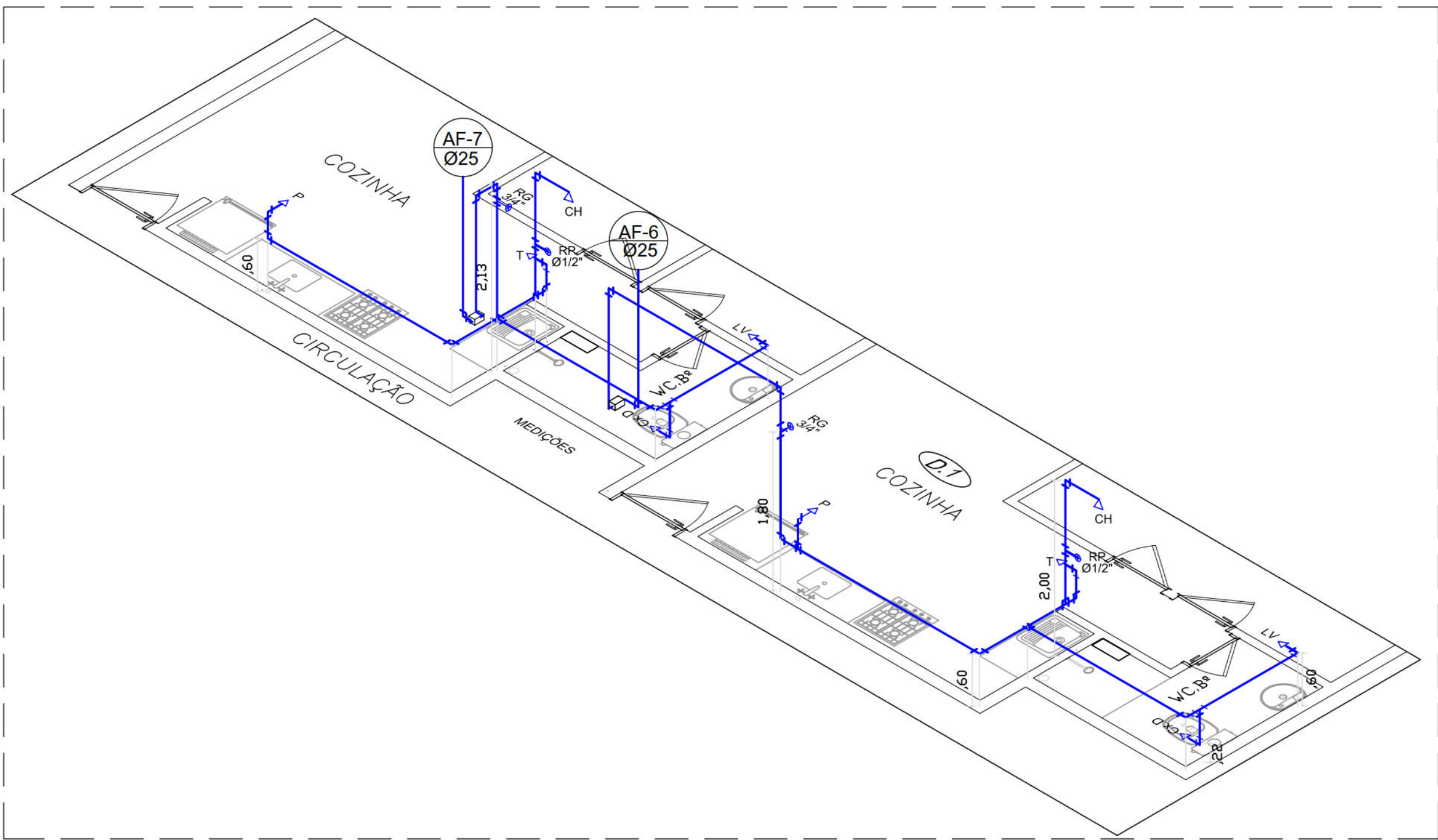
ISOMETRIA 1 ( PLANTA BAIXA - TÉRREO ) ESCALA: 1/50
