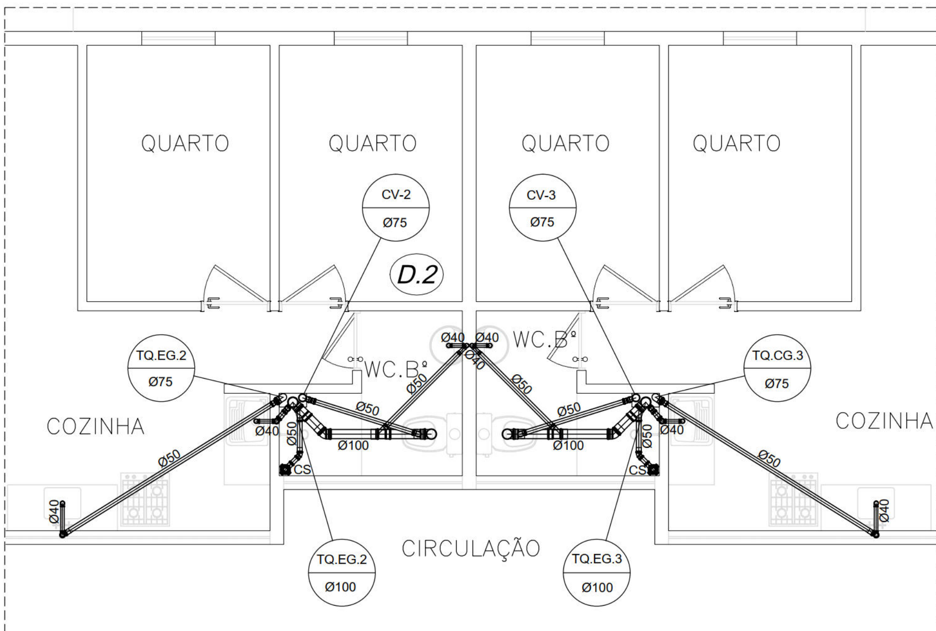
PLANTA BAIXA ESGOTO - 3º PAVIMENTO ESCALA: 1/25
