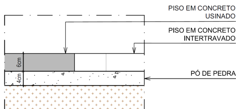
Figura 15 - Seção Tipo de Pavimentação
