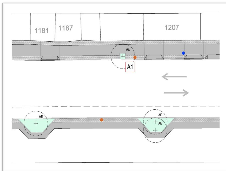
Figura 2 - Criação de novo passeio em área interna ao Parque - Planta de Proposta
