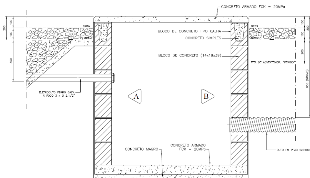
CORTE TRANSVERSAL
