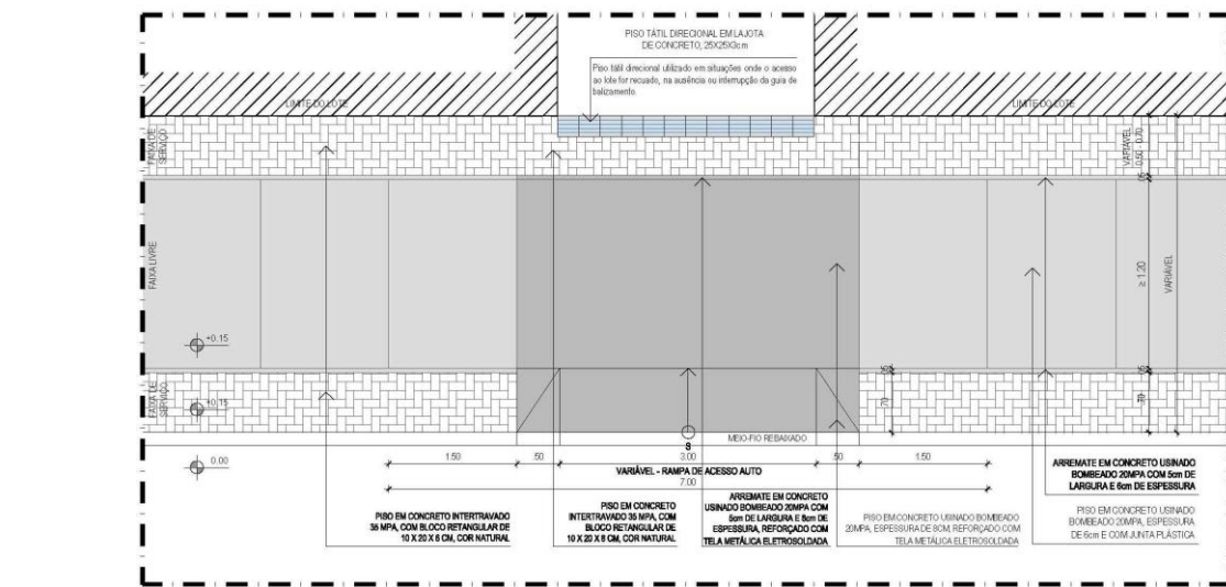
Figura 5 - Rampa padrão para o acesso de veículos
