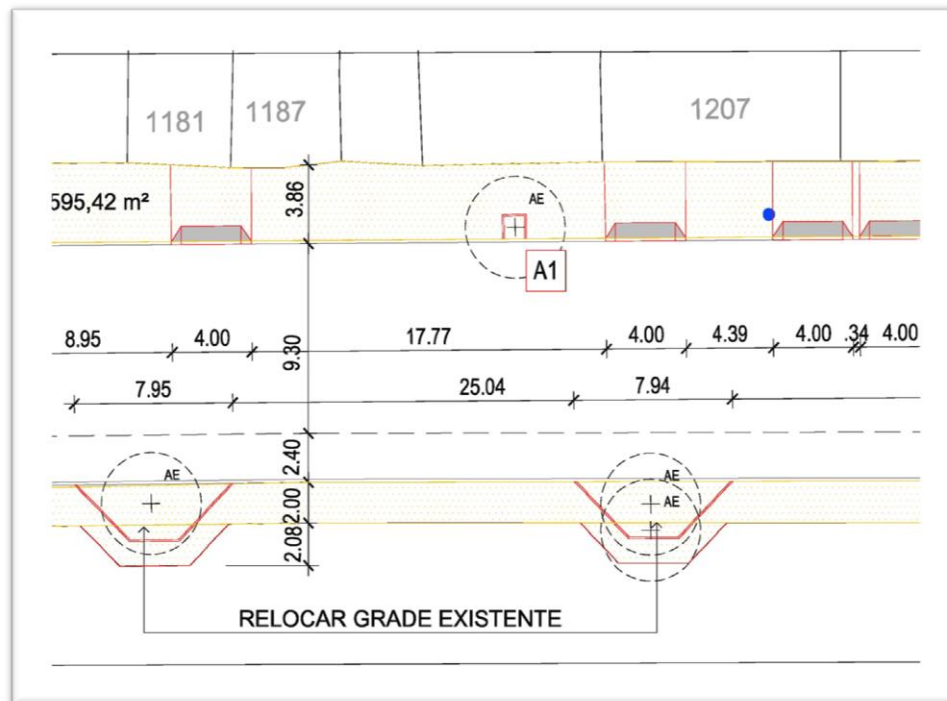
Figura 1 - Criação de novo passeio em área interna ao Parque - Planta de Reforma
